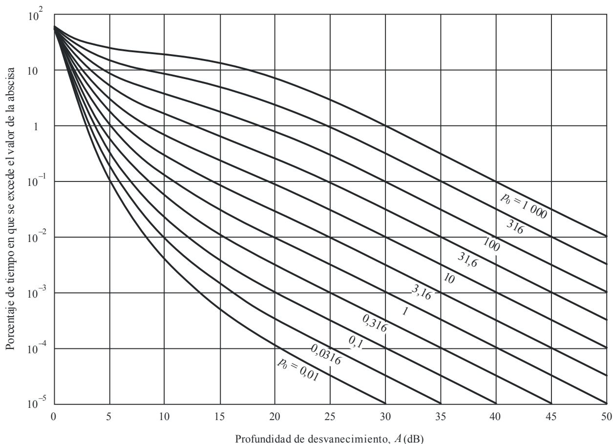
FIGURA 3 Porcentaje del tiempo, p_w , en que se excede la profundidad del desvanecimiento, A , en un mes más desfavorable medio para valores de p_0 (de la ecuación (10) o la (11), según sea el caso) comprendidos entre 0,01 y 1 000
