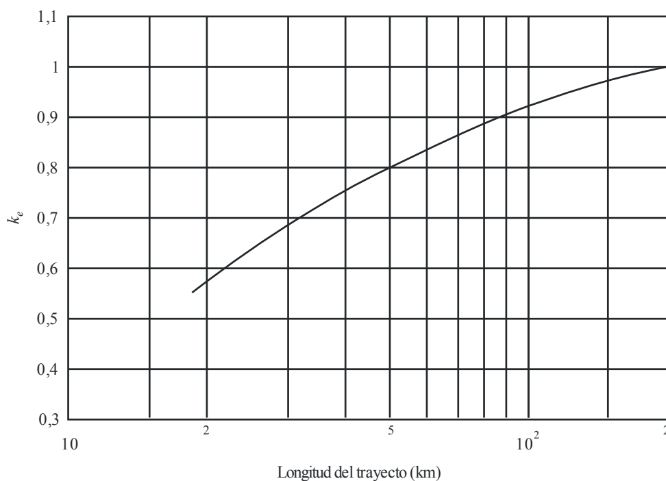
FIGURA 2 Valor de k_e excedido aproximadamente durante el 99,9% del tiempo (clima templado continental)
