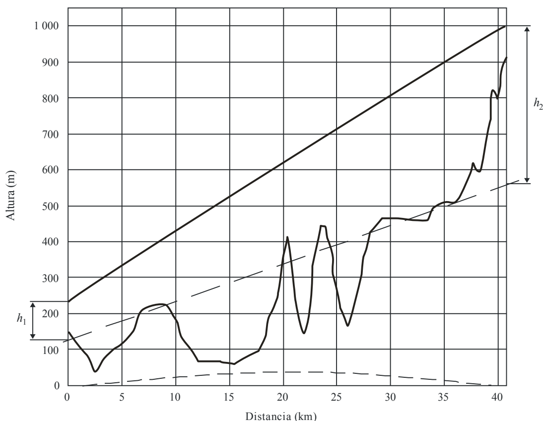
FIGURA 9 Trayecto con terreno reflectivo
