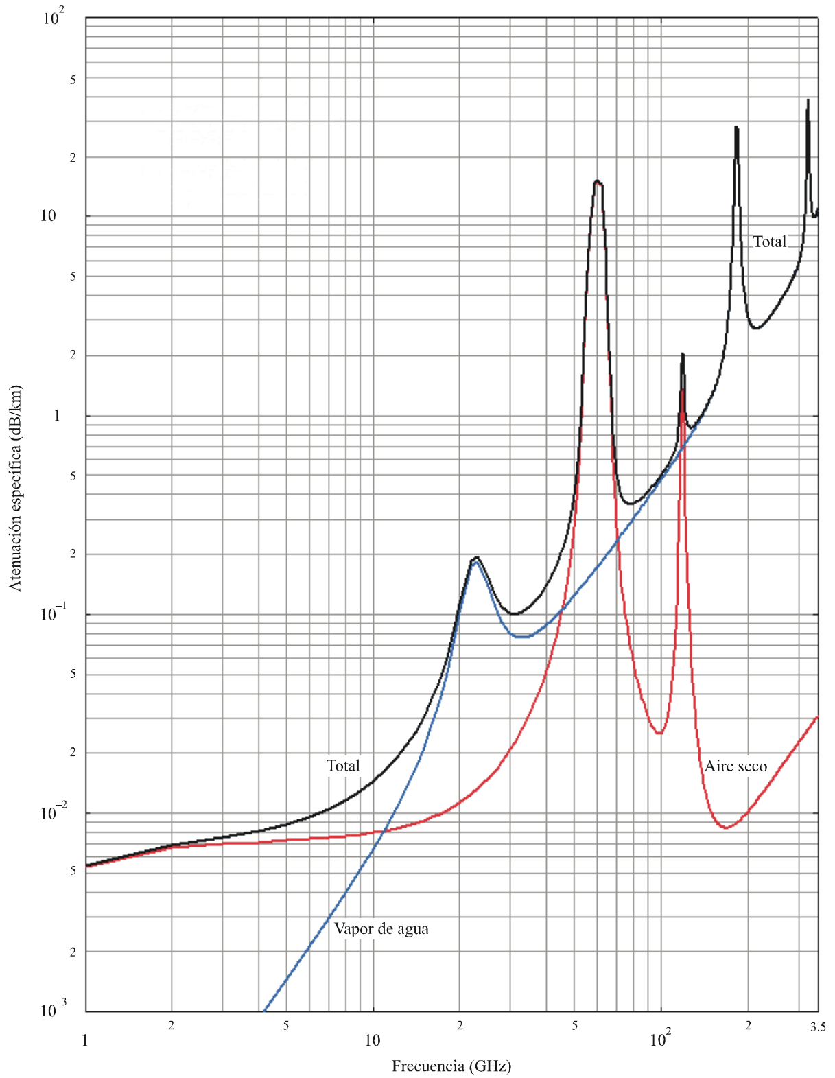
FIGURA 5 Atenuación específica debida a los gases
