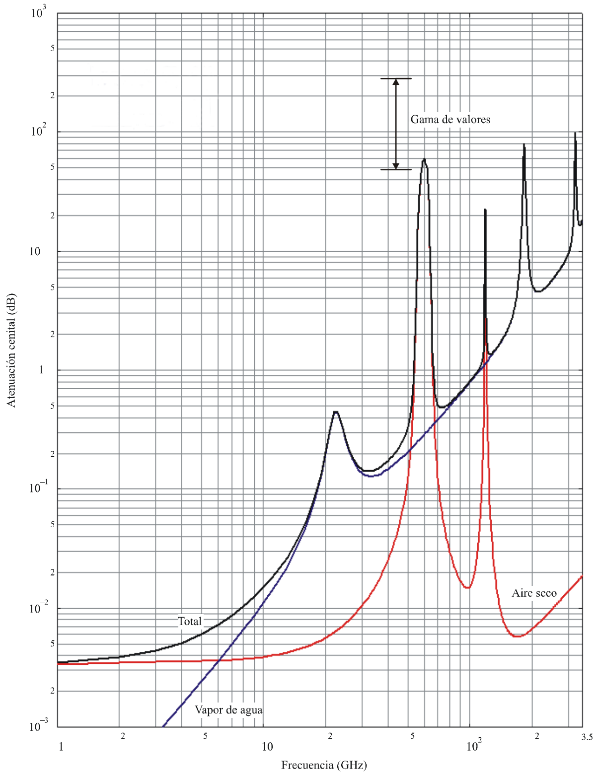
Atenuación cenital total a nivel del mar debida a la atmósfera seca y al vapor de agua
