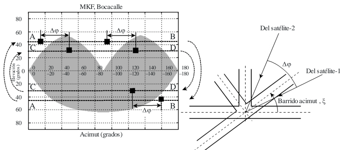
Cálculo de la disponibilidad total del sistema para una constelación de satélites OSG con respecto a una bocacalle
