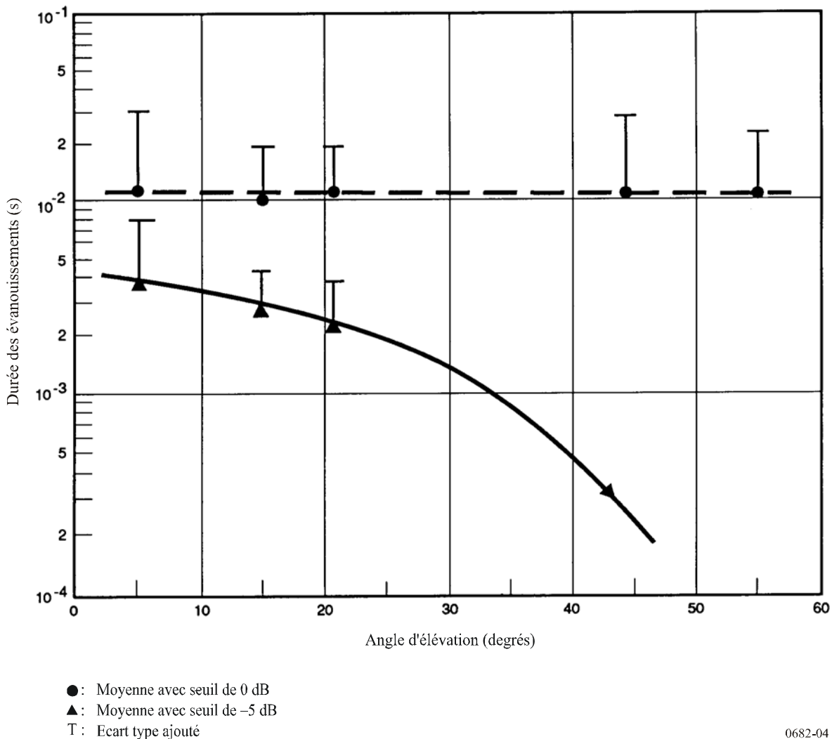
FIGURE 4 Durée des évanouissements en fonction de l'angle d'élévation pour une polarisation circulaire à 1,6 GHz (gain d'antenne = 3,5 dBi); données obtenues au-dessus de l'Atlantique et de l'Europe occidentale
