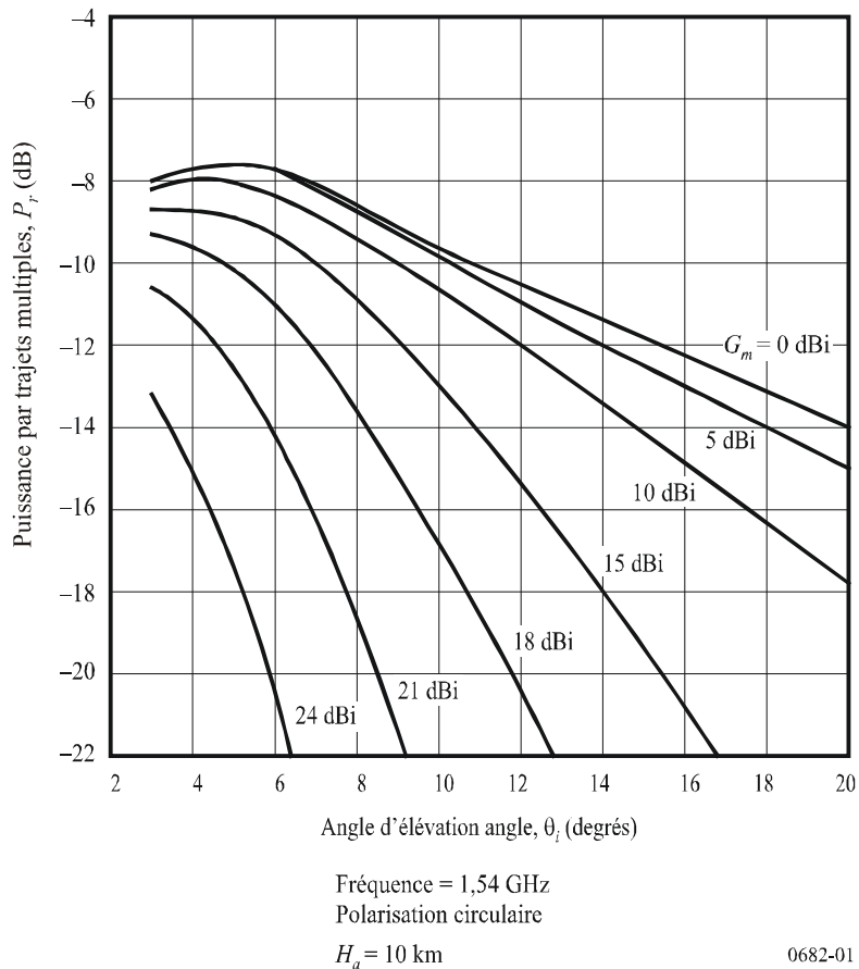
FIGURE 1 Puissance moyenne par trajets multiples relative à la puissance du signal direct, en fonction de l'angle d'élevation pour différents gains d'antenne
