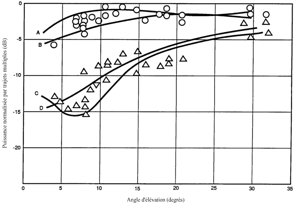
FIGURE 3 Puissance normalisée par trajets multiples au-dessus de l'océan en fonction de l'angle d'élévation à 1,6 GHz
