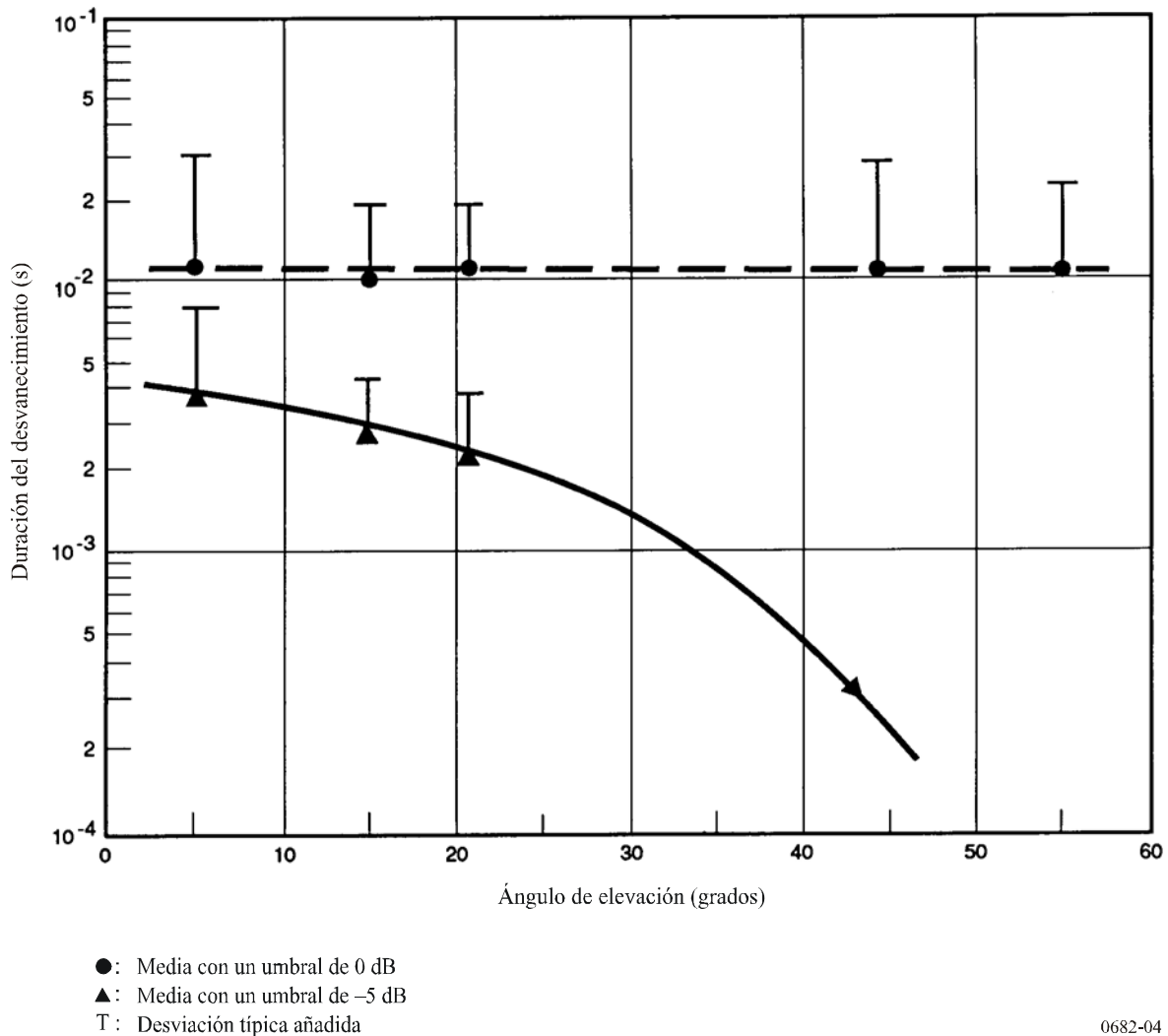
FIGURA 4 Duración del desvanecimiento en función del ángulo de elevación para polarización circular a 1,6 GHz (ganancia de antena = 3,5 dBi), datos recogidos sobre el Océano Atlántico y Europa occidental
