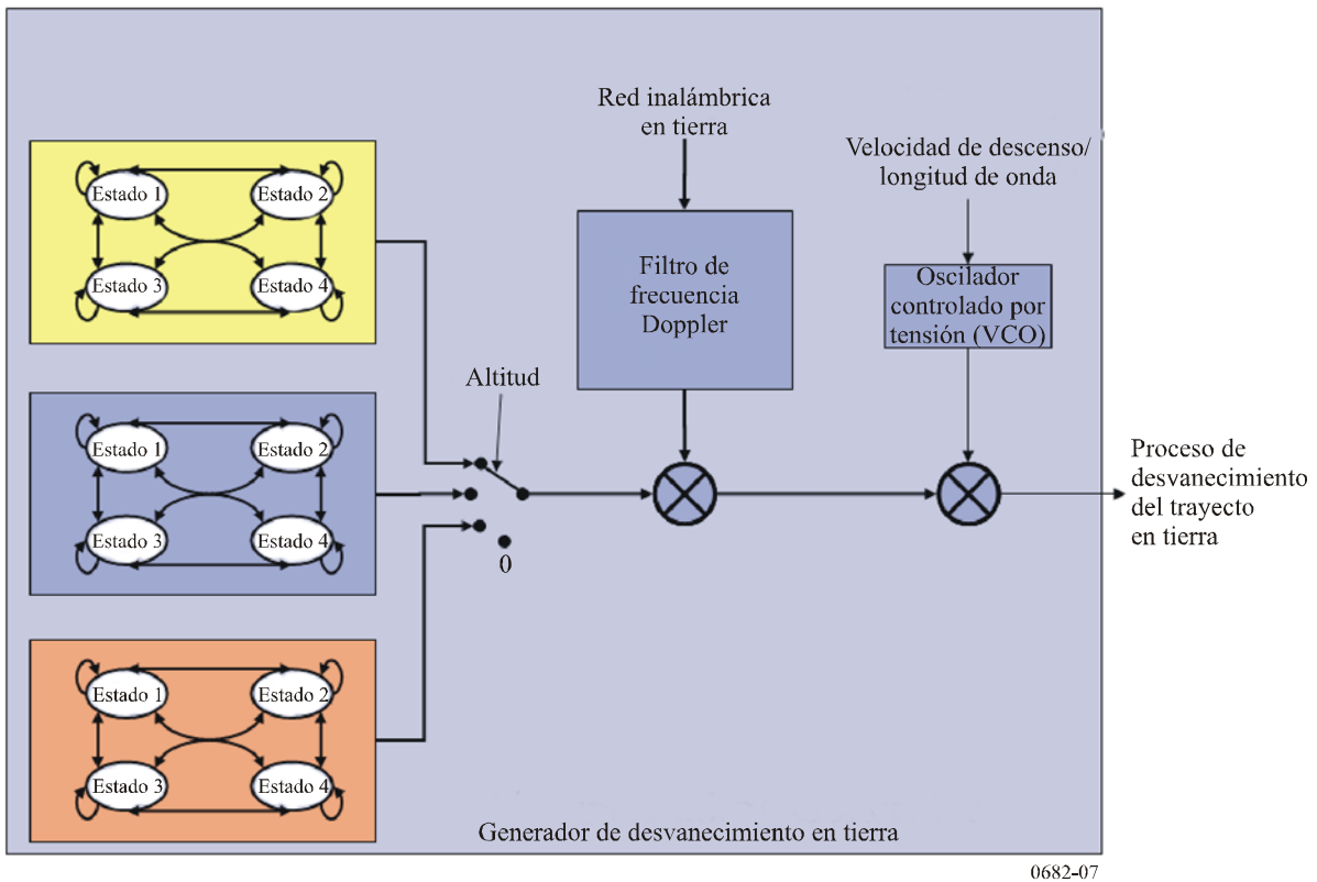
FIGURA 7 Esquema de un módulo generador de desvanecimiento en tierra
