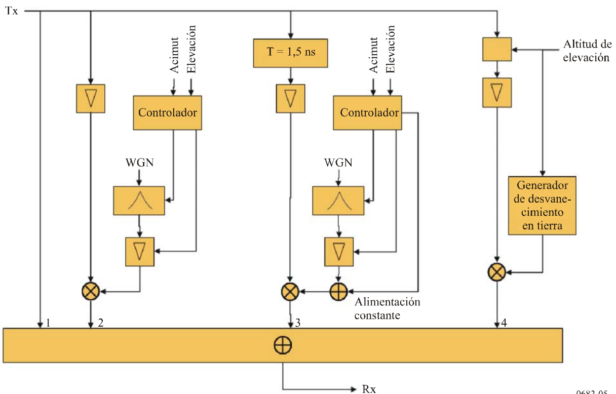
FIGURA 5 Modelo de canal aeronáutico completo
