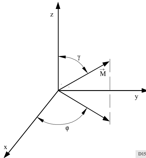
FIGURA 15 Orientación del dipolo \vec{M} dentro del guíaondas, siendo \gamma la inclinación y \phi la orientación acimutal
