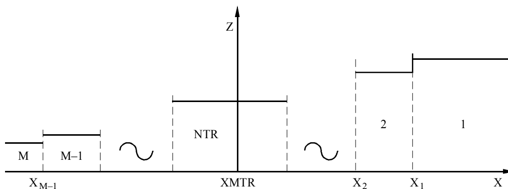
FIGURA 16 Modelo de conversión de modos
