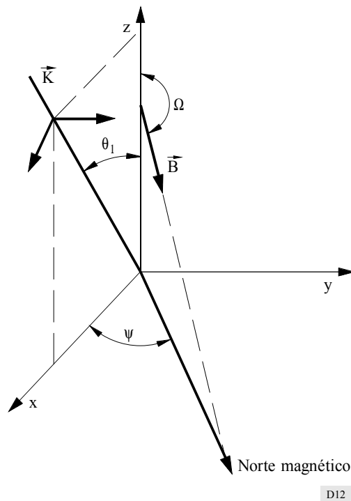
FIGURA 12 Geometría de propagación de las ondas
