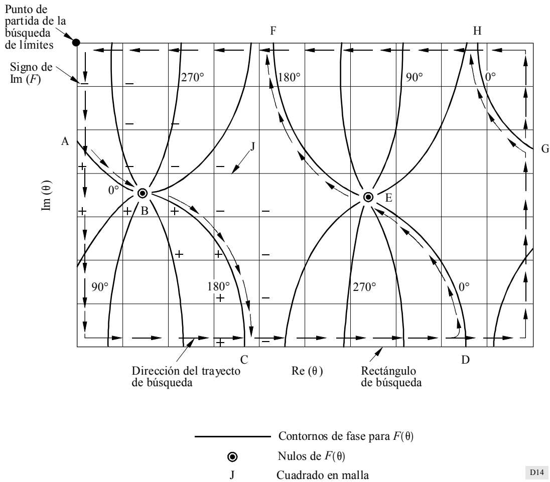
FIGURA 14 Método para hallar los modos para la función F(\theta)
