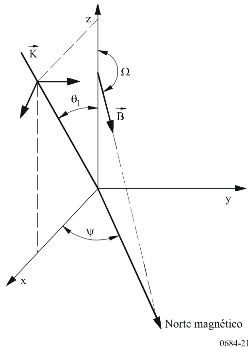
FIGURA 21 Geometría de propagación de las ondas
