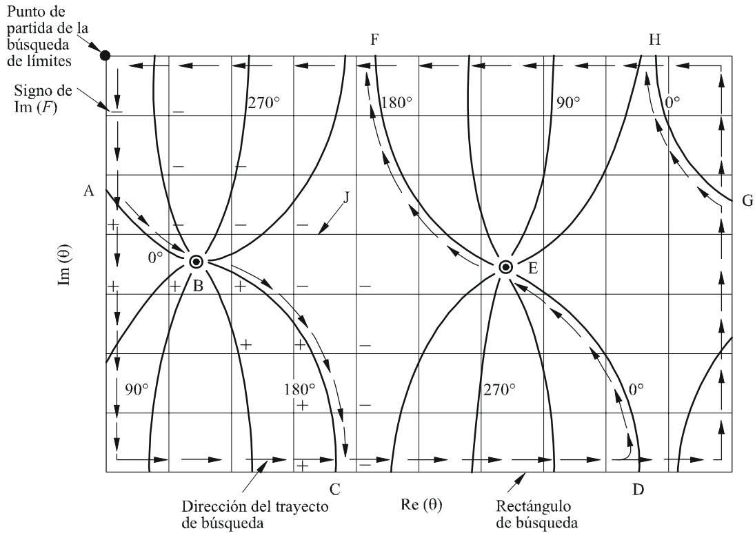
FIGURA 23 Método para hallar los modos para la función F(\theta)
