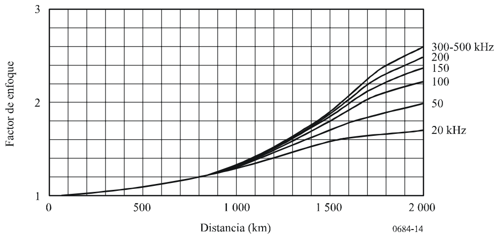
FIGURA 14 Factor de enfoque
