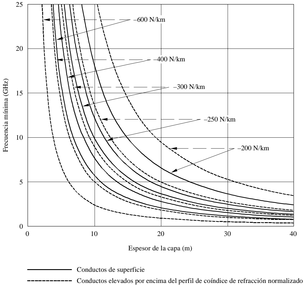
FIGURA 3 Frecuencia mínima en conductos radioeléctricos atmosféricos de gradiente de coíndice constante
