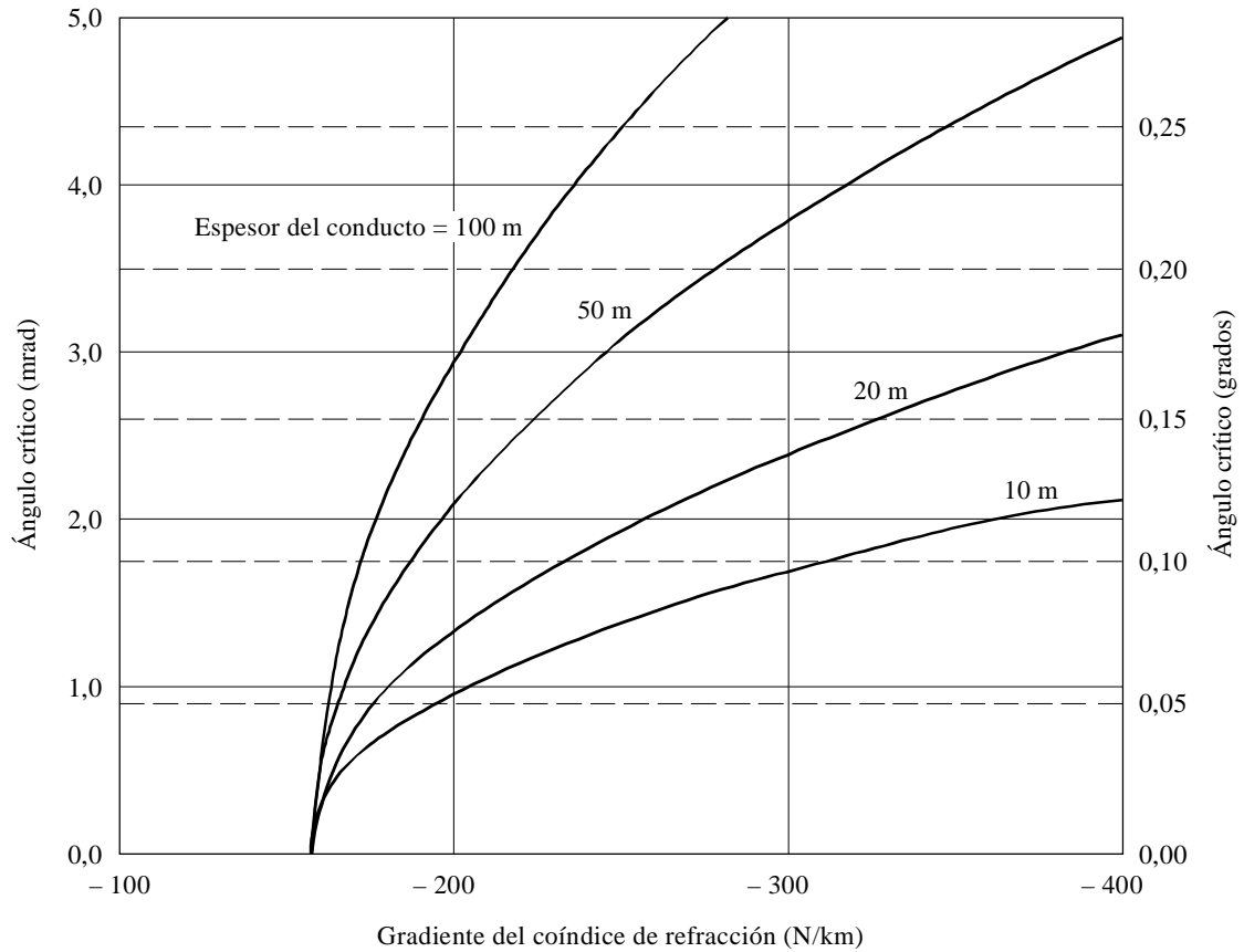
FIGURA 2 Ángulo máximo para un conducto de superficie de gradiente de coíndice constante sobre una tierra esférica
