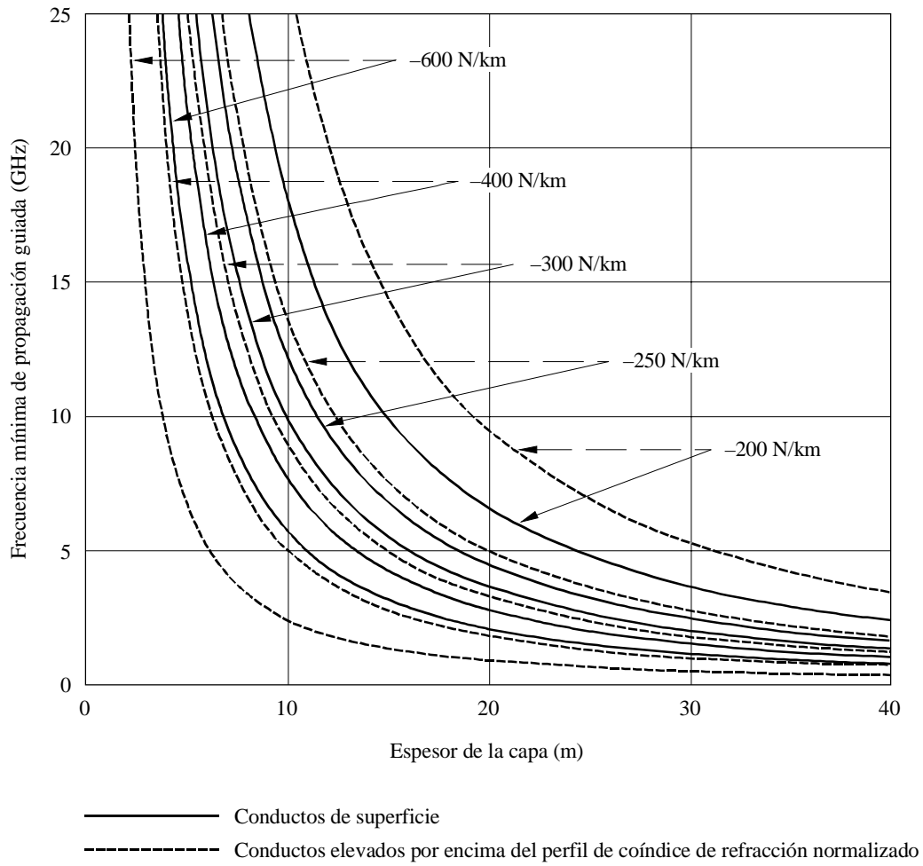
FIGURA 4 Frecuencia mínima de propagación guiada para conductos radioelétricos atmosféricos de gradiente de coíndice constante
