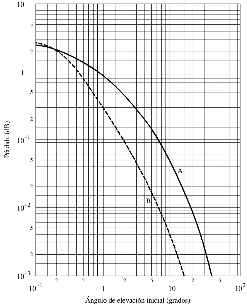
FIGURA 1 Estimación de la pérdida debida a la dispersión adicional de un haz y desviación típica con respecto a la media
