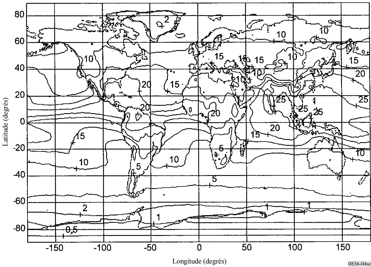
FIGURE 4 Juin, juillet, août: concentration en vapeur d'eau à la surface de la Terre ( \text{g}/\text{m}^3 )
