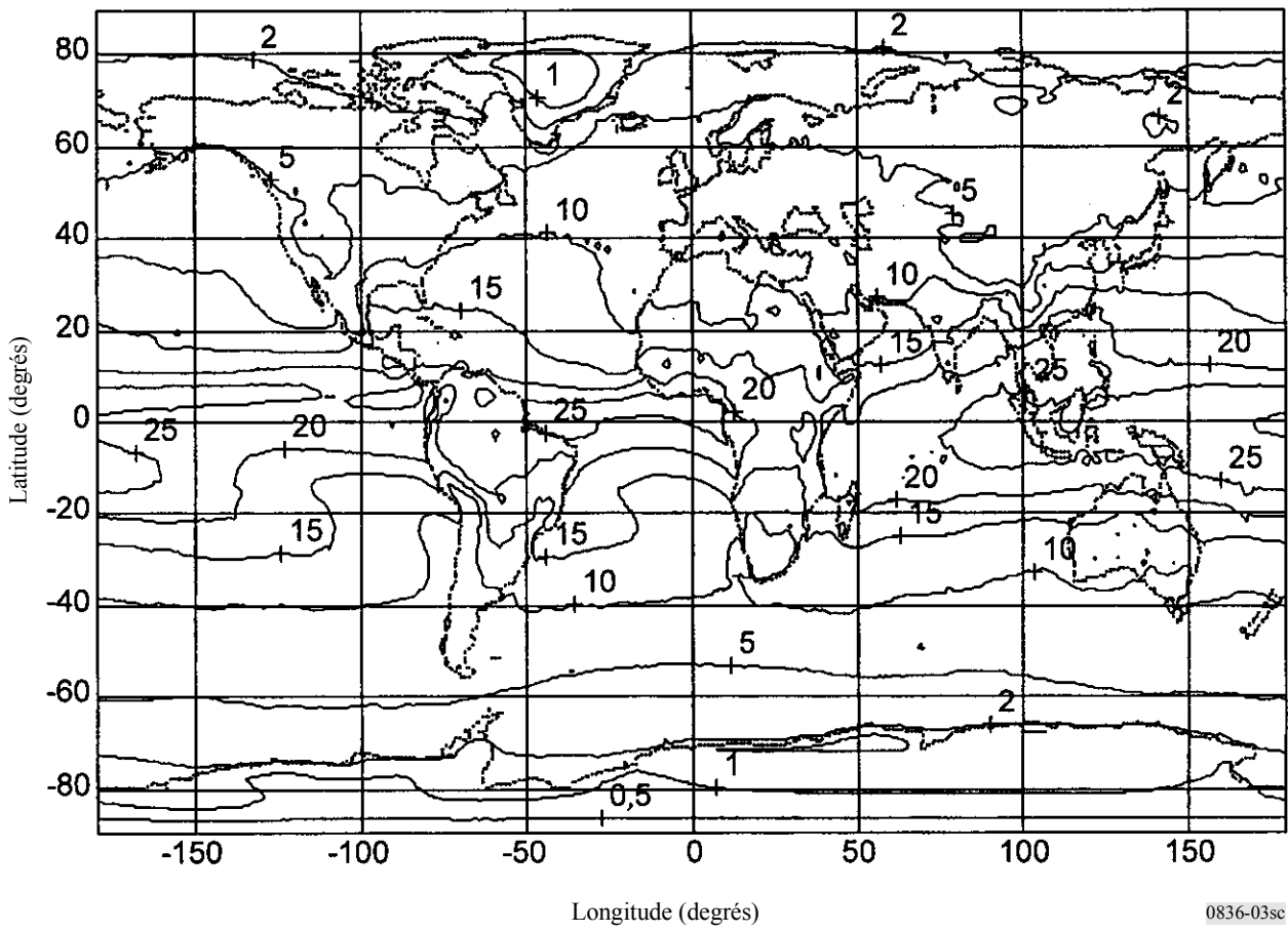
FIGURE 3 Mars, avril, mai: concentration en vapeur d'eau à la surface de la Terre ( \text{g}/\text{m}^3 )
