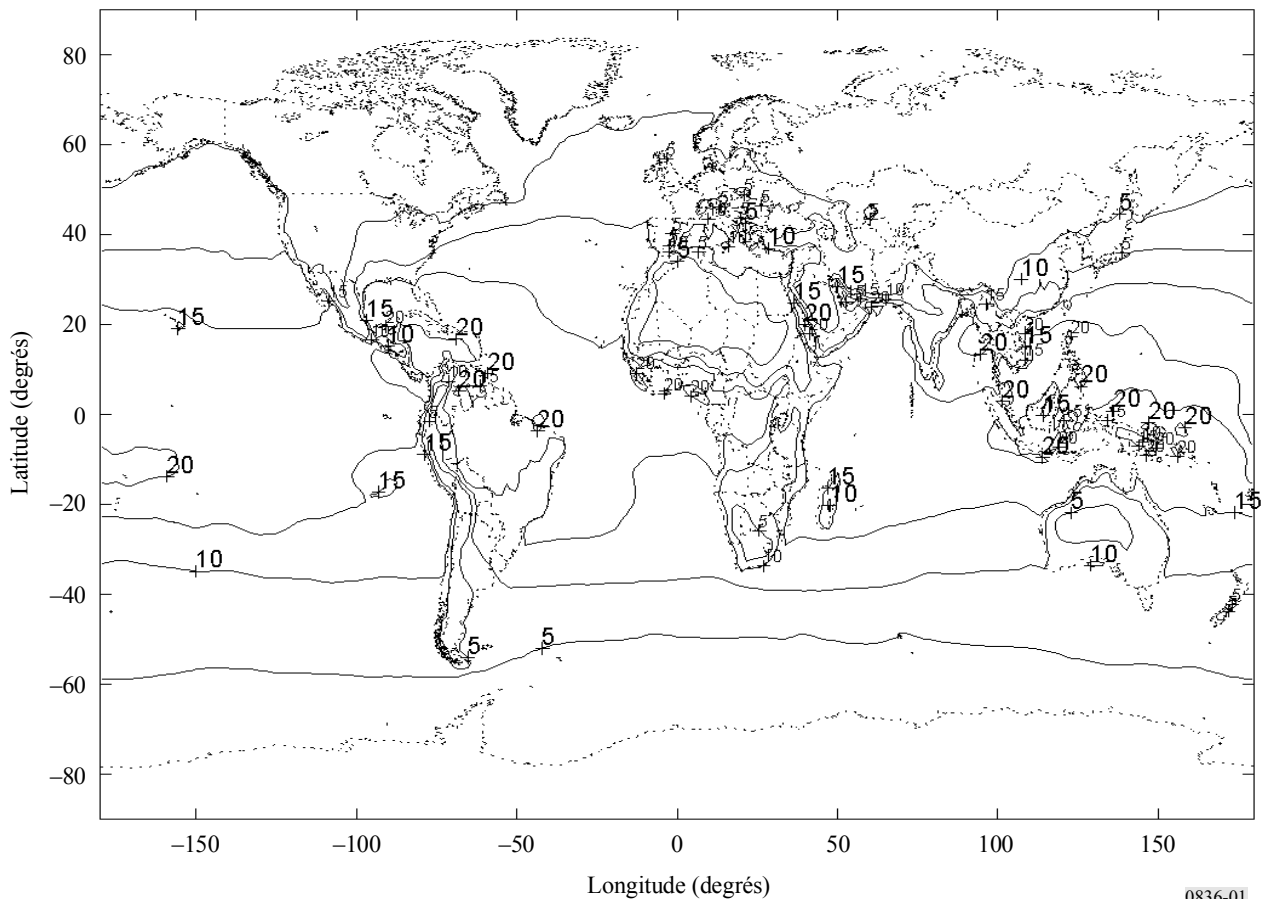
FIGURE 1 Concentration en vapeur d'eau à la surface de la Terre ( \text{g}/\text{m}^3 ) dépassée pendant 50% de l'année
