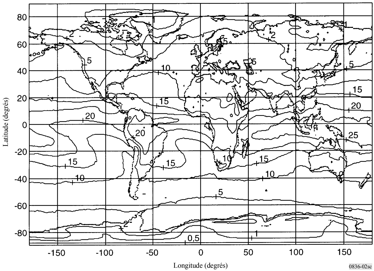
FIGURE 2 Décembre, janvier, février: concentration en vapeur d'eau à la surface de la Terre (g/m 3 )
