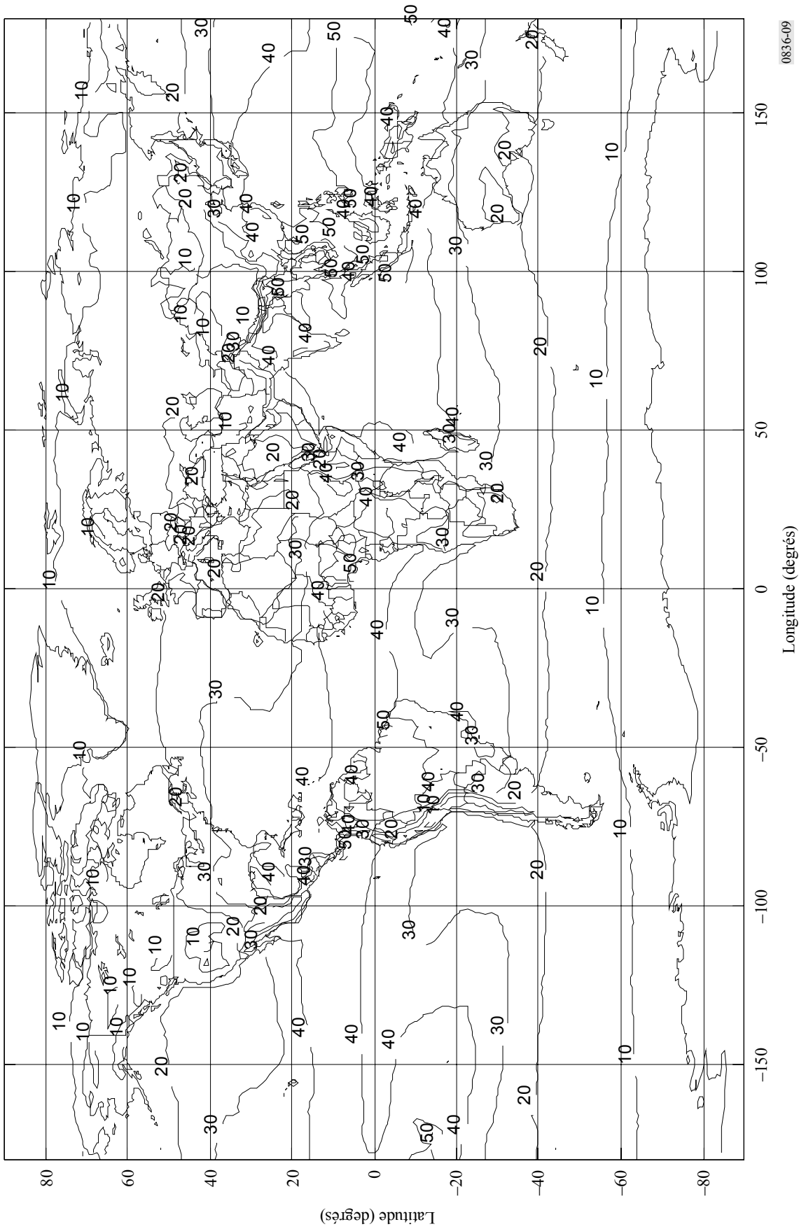
FIGURE 9 Colonne d'air en vapeur d'eau (kg/m 3 ), valeur dépassée pendant 20% de l'année
