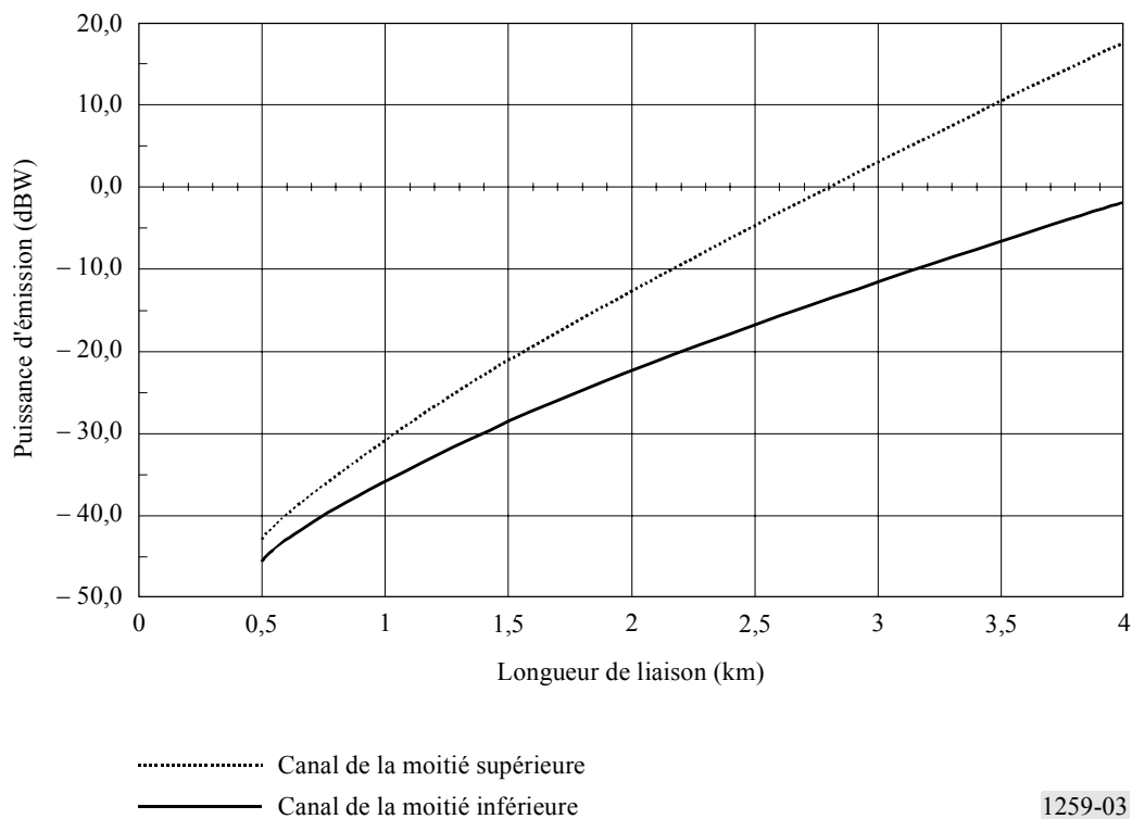
FIGURE 3 Puissance d'émission en fonction de la longueur des liaisons
