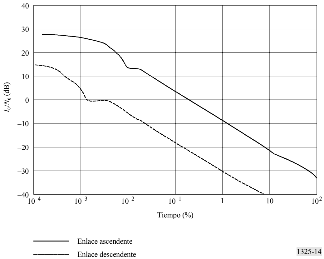
FIGURA 14 Interferencia causada por una red OSG a un sistema no OSG
