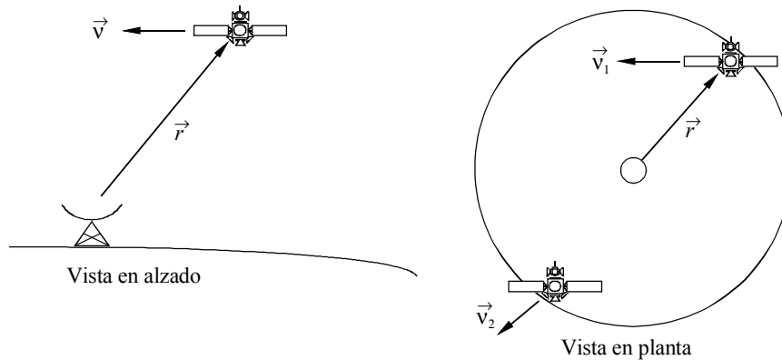
FIGURA 4 Criterio de selección de la siguiente estación espacial desde la estación terrena para establecer un enlace de comunicaciones
