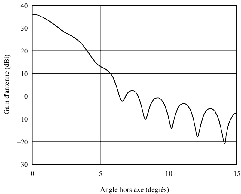
FIGURE 9 Diagramme de gain d'antenne à faisceaux ponctuels USAKUM3 (émission et réception)
