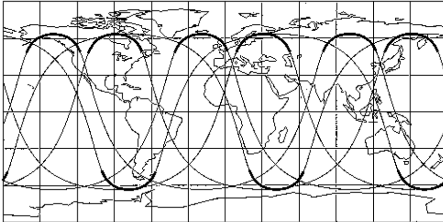
Trajectoires au sol des points subsatellite du système USAKU-H2
