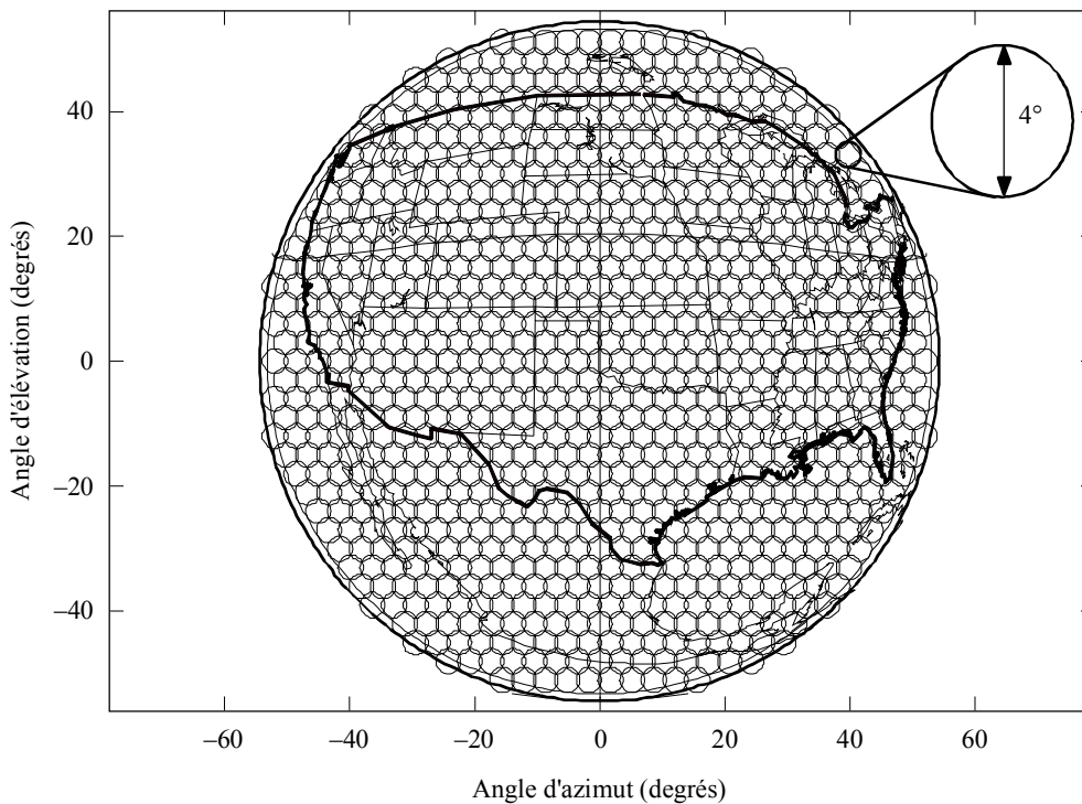
FIGURE 6 Couverture par faisceaux ponctuels USAKUL2 (émission et réception)
