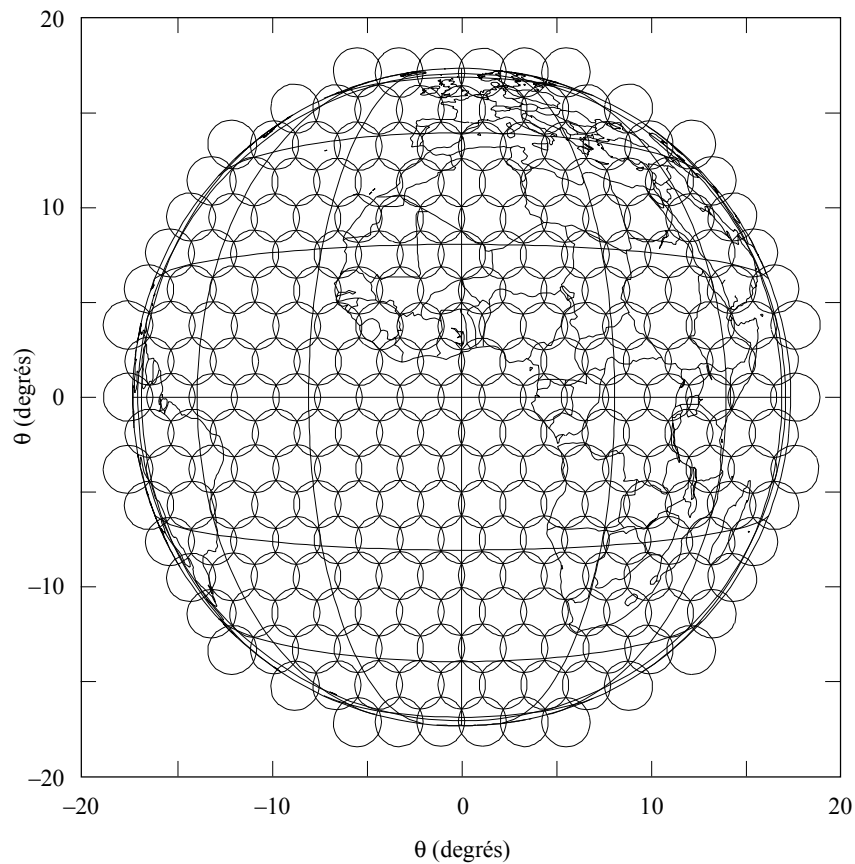
FIGURE 8 Couverture par faisceaux ponctuels USAKUM3 (émission et réception)
