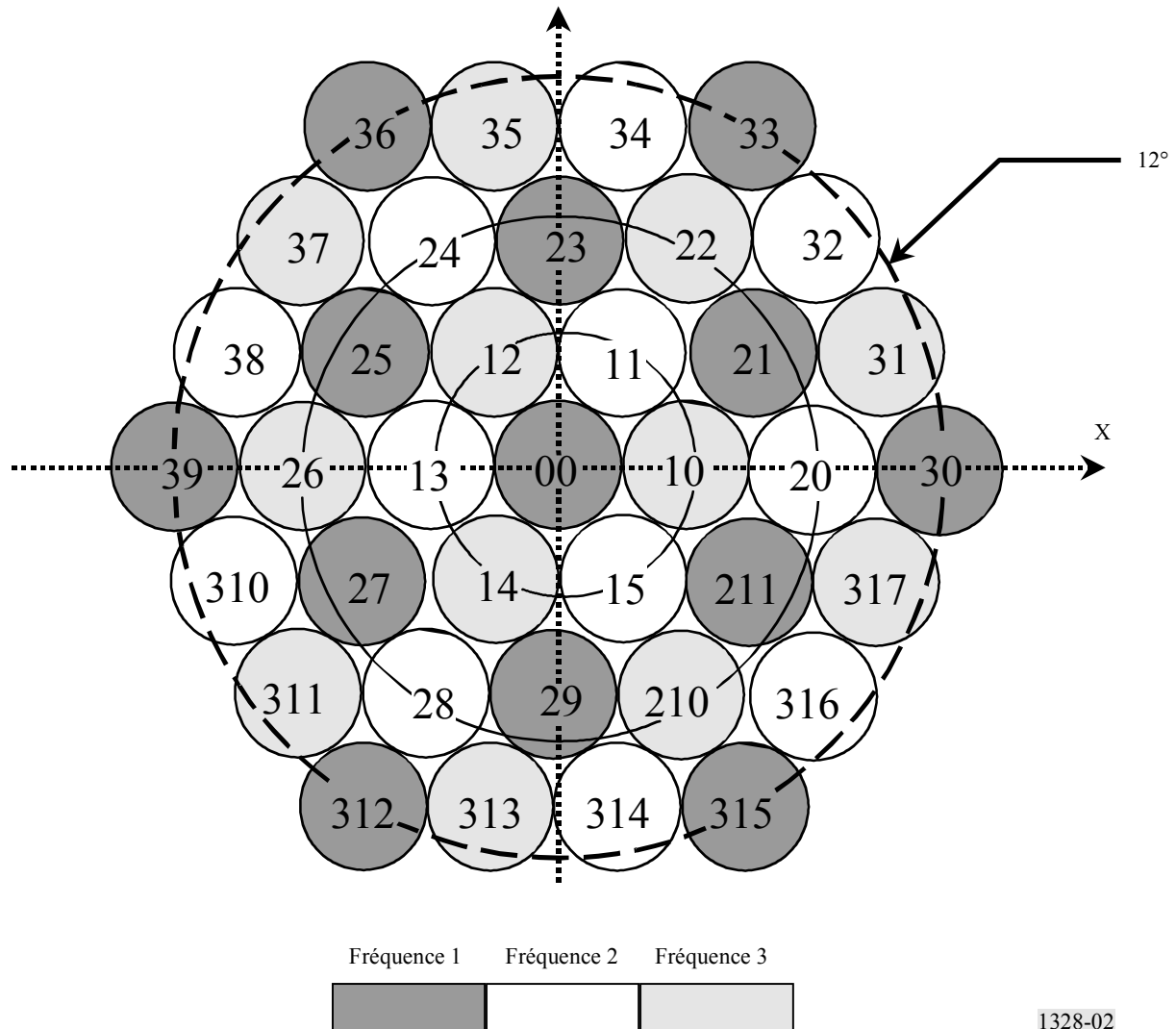
FIGURE 2 Schéma de réutilisation des fréquences et des polarisations
