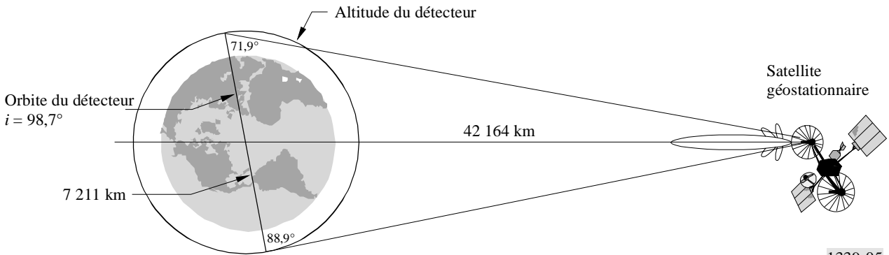
FIGURE 5 Géométrie du second cas Vue du plan de l'équateur
