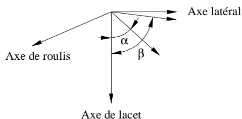
FIGURE 1 Plan de balayage du détecteur passif
