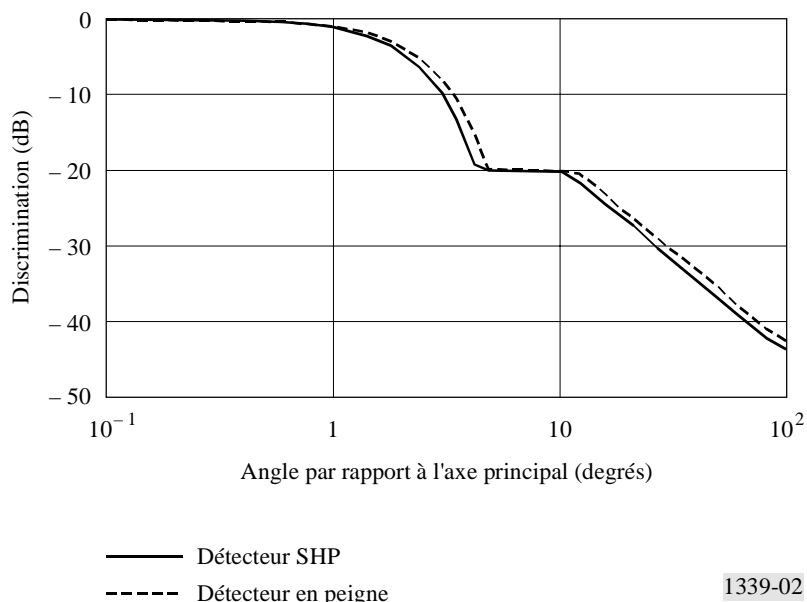
FIGURE 2 Diagrammes d'antenne d'étalonnage de détecteur
