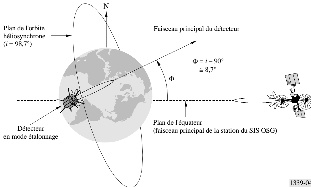
FIGURE 4 Détecteur passif dans le plan de l'équateur
