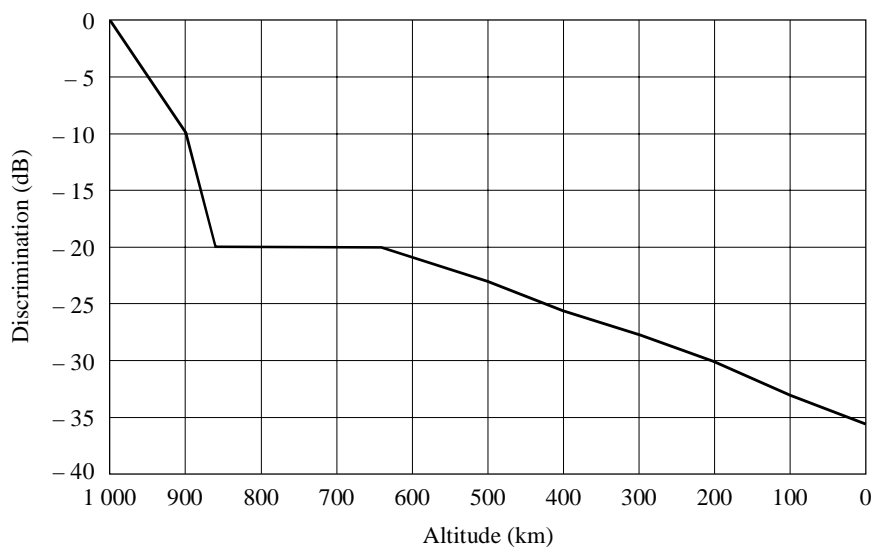
FIGURE 12 Discrimination d'un système SIS OSG type depuis 1 000 km (Puissance surfacique maximale à 1 000 km)
