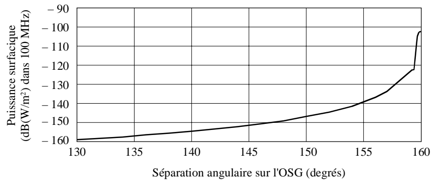
FIGURE 3 Séparation angulaire permise sur l'OSG en fonction de diverses limites de puissance surfacique
