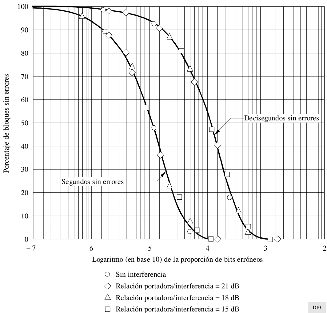
FIGURA 8 Distribución de bloques sin errores: 64 kbit/s, sin codificación FEC
