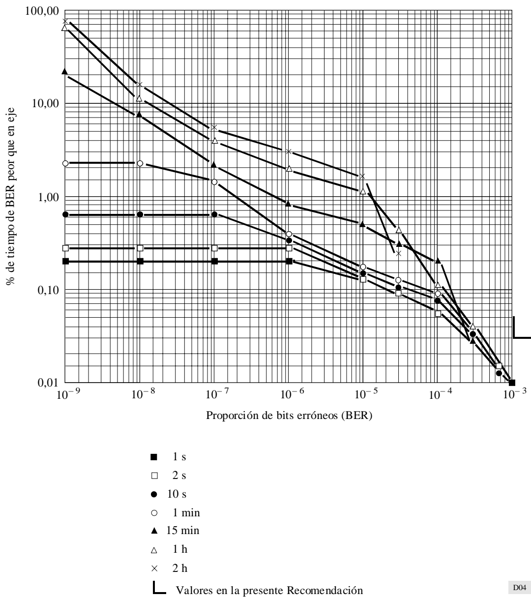
FIGURA 4 Examen de la relación existente entre los valores medidos de BER y los valores de las mediciones de los parámetros de la Recomendación UIT-T G.821
