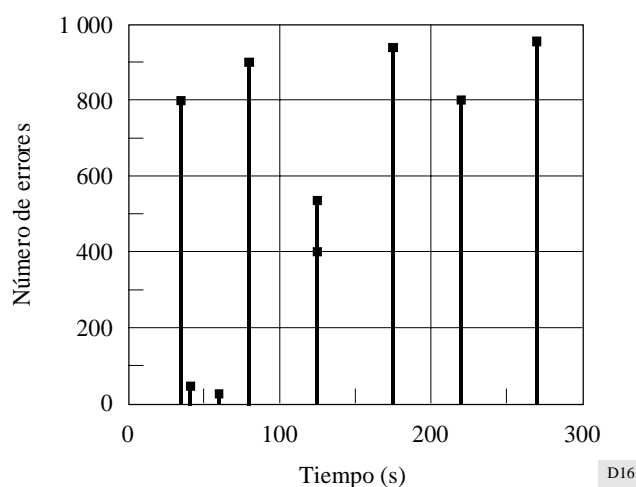
FIGURA 13 Distribución de errores en la salida del decodificador secuencial
