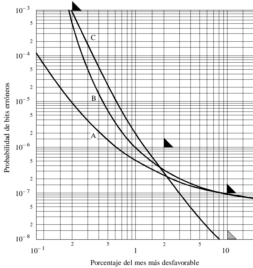
FIGURA 21 Características de un sistema que funciona en las bandas 14/11 GHz diseñado para cumplir exactamente los objetivos de esta Recomendación
