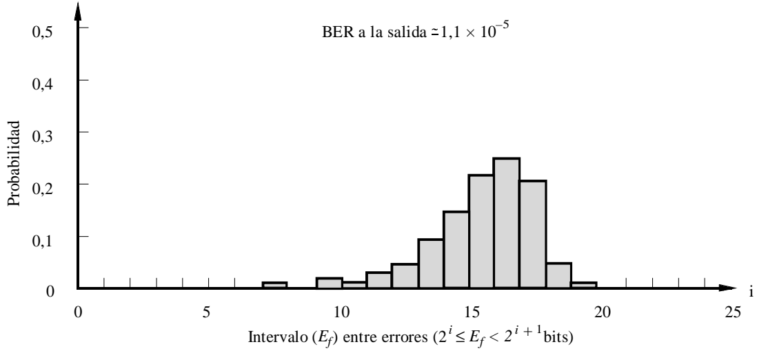
FIGURA 9 Distribución de errores con y sin FEC
