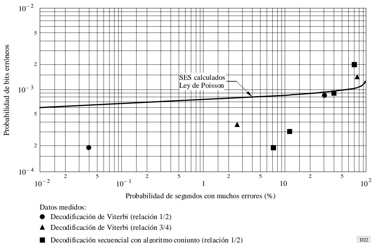
FIGURA 19 Probabilidad de segundos con muchos errores (SES) para un tren binario a 64 kbit/s
