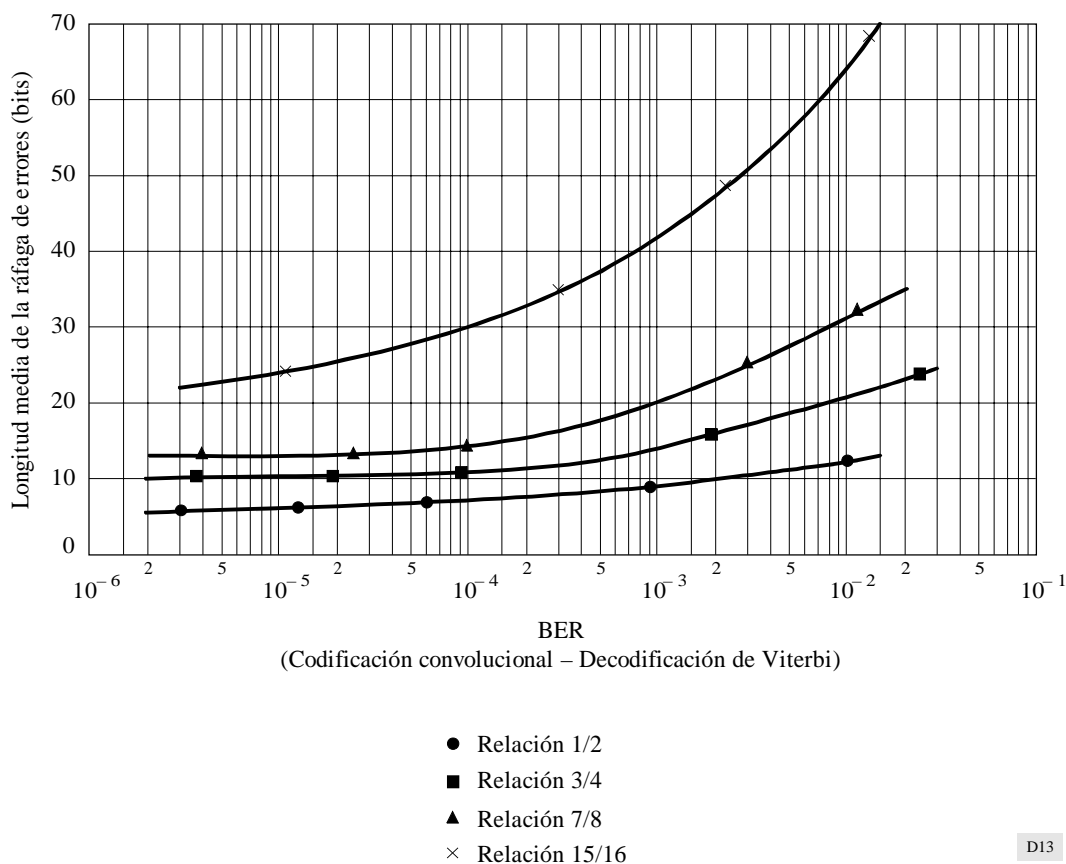
FIGURA 11 Distribución entre la longitud media de los errores en ráfaga y la BER
