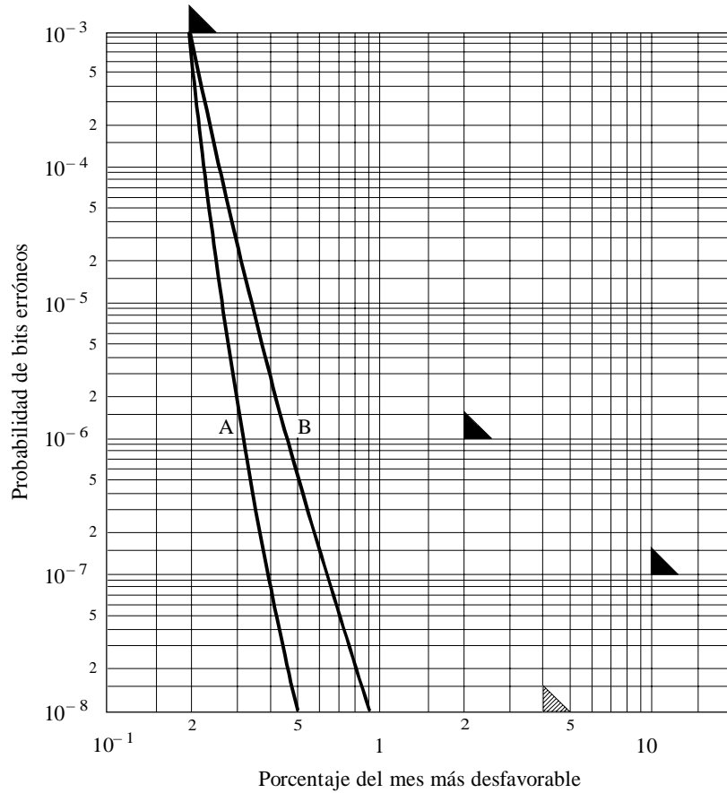
FIGURA 22 Características de un sistema que funciona en las bandas 14/11 GHz diseñado para cumplir exactamente los objetivos de esta Recomendación
