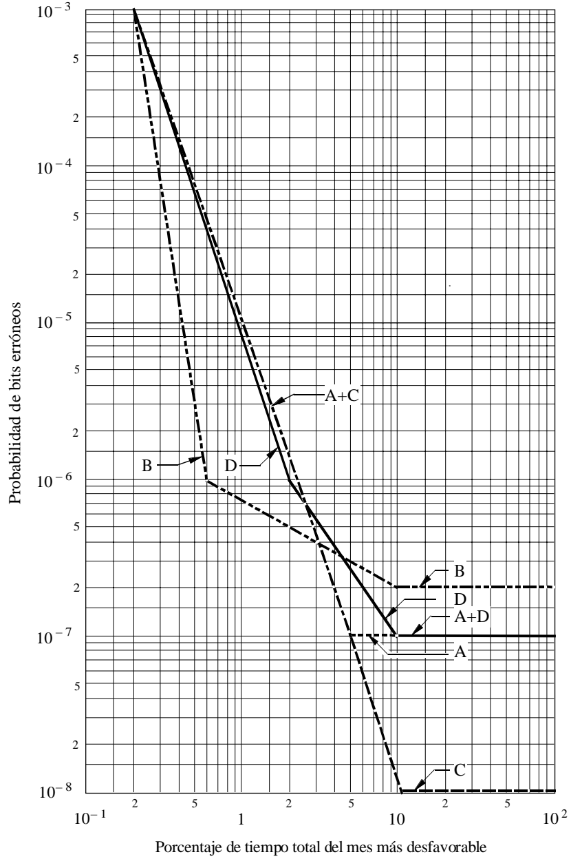
FIGURA 3 Modelos de PEB que se ajustan a la Recomendación UIT-T G.821
