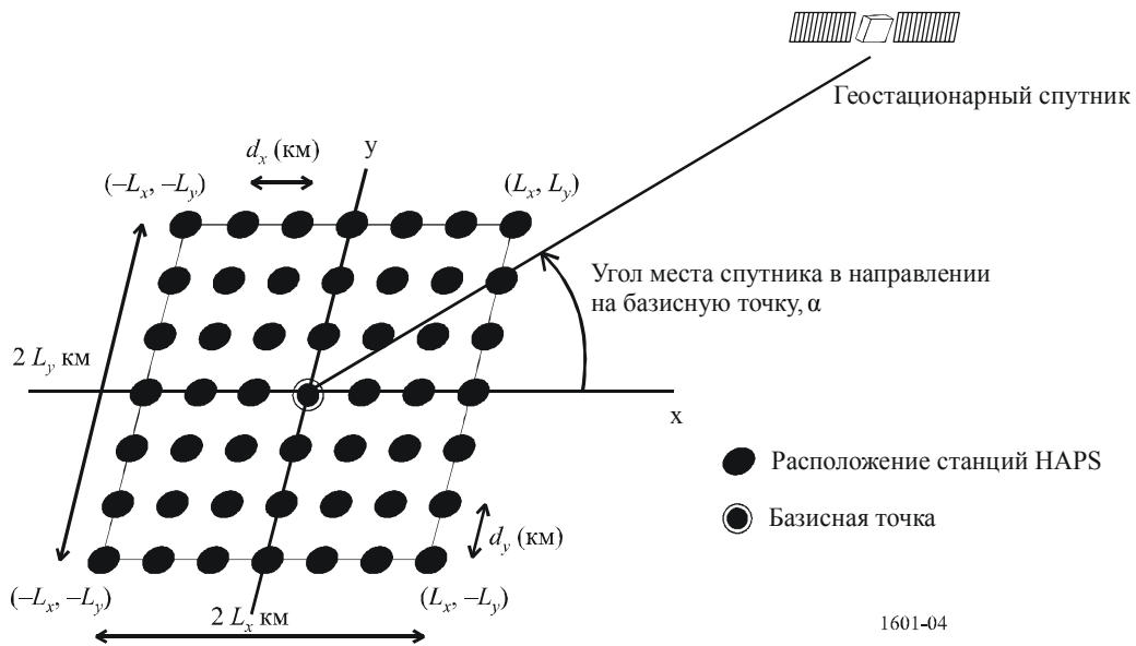
Модель развертывания системы HAPS
