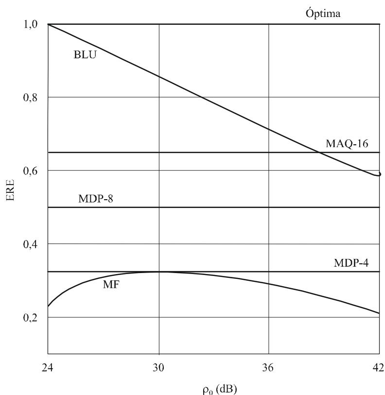
FIGURA 2 ERE en una red con diferentes tipos de modulación
