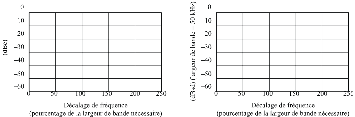
FIGURE 10 Exemples de l'étiquetage préféré de l'axe des Y pour les gabarits symétriques des émissions hors bande, utilisant les niveaux relatifs
