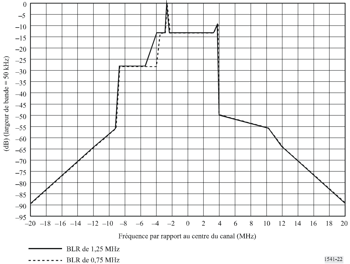
FIGURE 22 Gabarit de limite spectrale pour la télévision analogique à 8 MHz, modulation positive (pour P = 39 à 50 dBW)
