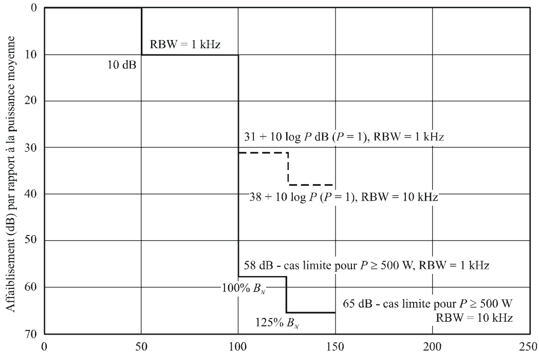
FIGURE 38 Stations fonctionnant au-dessus de 30 MHz dans le cas à large bande de la Recommandation UIT-R SM.1539
