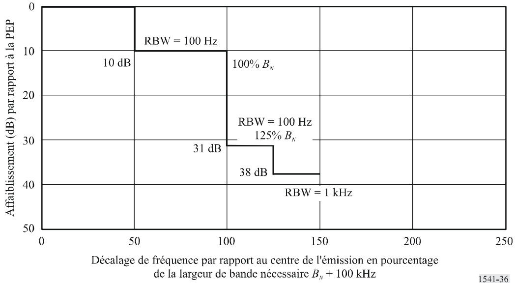
FIGURE 36 Stations fonctionnant au-dessous de 30 MHz dans le cas à large bande de la Recommandation UIT-R SM.1539
