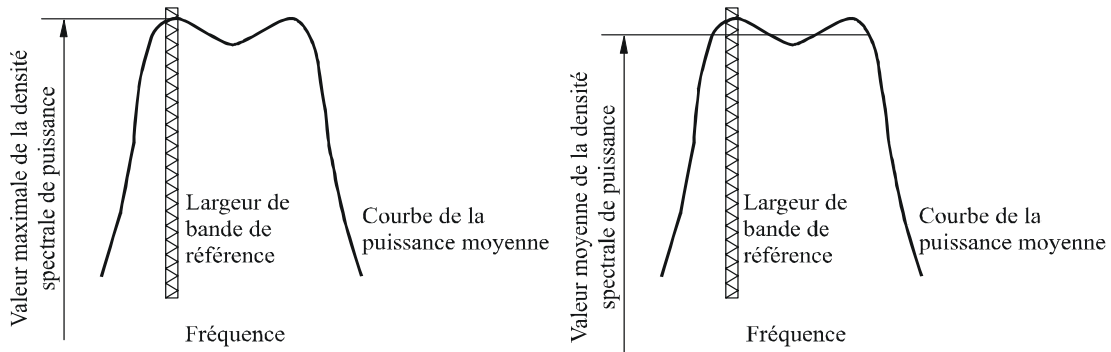
a) Concept de densité spectrale de puissance maximale b) Concept de densité spectrale de puissance moyenne
