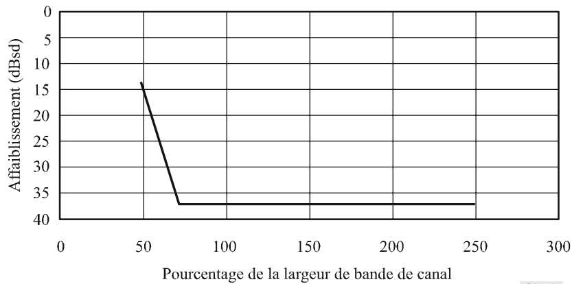
FIGURE 41 Gabarit des émissions hors bande pour les systèmes mobiles terrestres à largeur de bande de canal de 6,5 kHz
