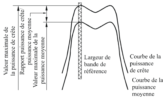
Concept de puissance de crête
