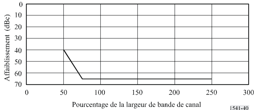
FIGURE 40 Gabarit des émissions hors bande pour les systèmes à BLU avec compression-extension d'amplitude et à largeur de bande de canal de 5 kHz
