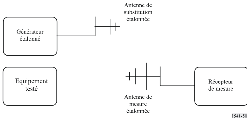
FIGURE 50 Montage simplifié pour la mesure de la p.i.r.e. des émissions dans le domaine des émissions hors bande
