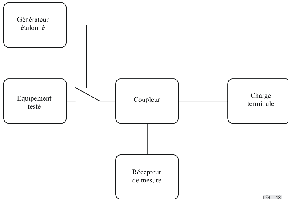
FIGURE 48 Montage simplifié pour la mesure de la puissance des émissions dans la bande et des émissions hors bande au niveau du port antenne
