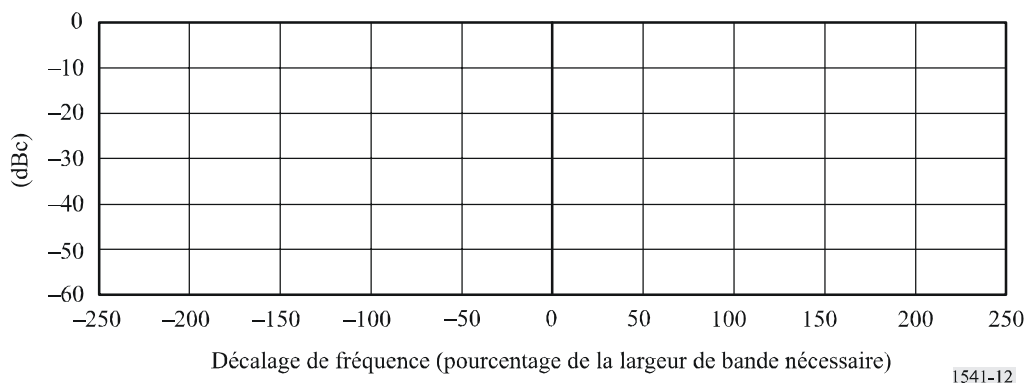
FIGURE 12 Exemple d'étiquetage pour des gabarits symétriques ou non des émissions hors bande
