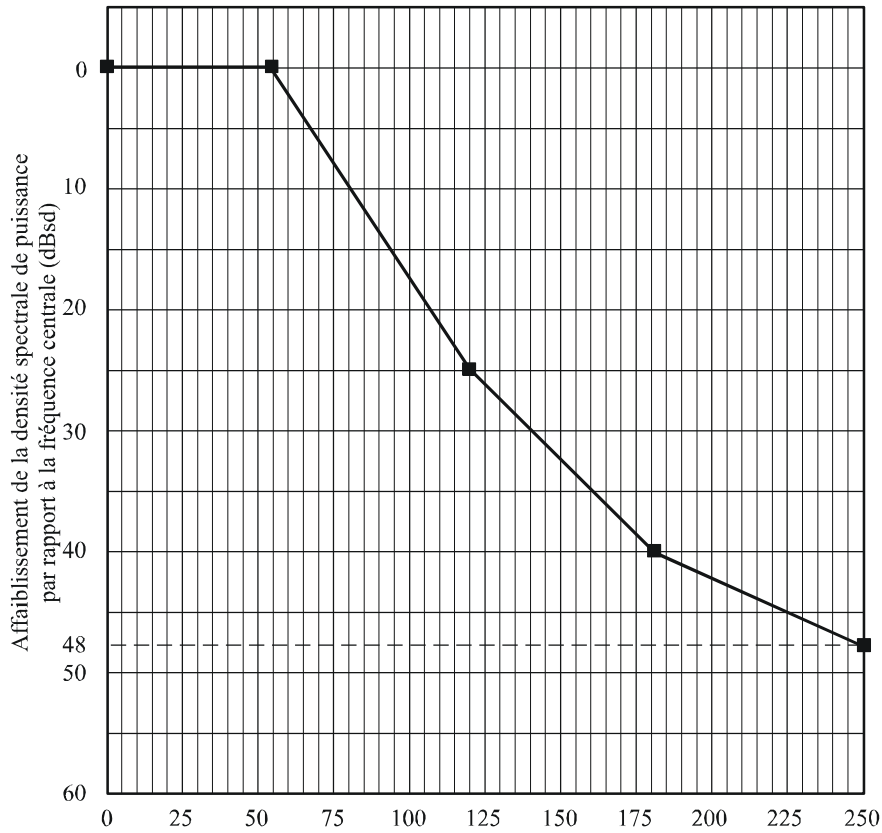
FIGURE 46 Gabarits spectraux génériques pour le service fixe numérique fonctionnant au-dessous de 30 MHz (Voir le Tableau 29)
