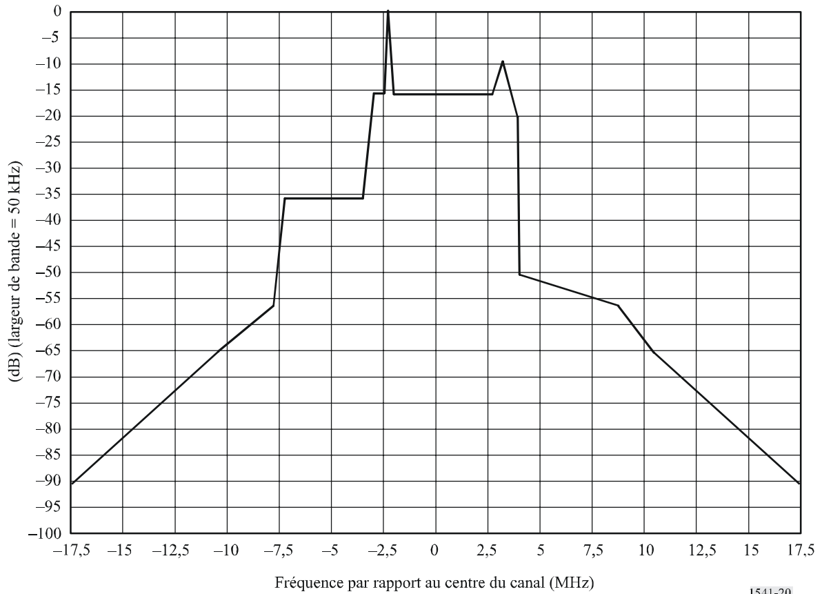
FIGURE 20 Gabarit de limite spectrale pour la télévision analogique à 7 MHz, modulation négative, BLR de 0,75 MHz (pour P = 39 à 50 dBW)
