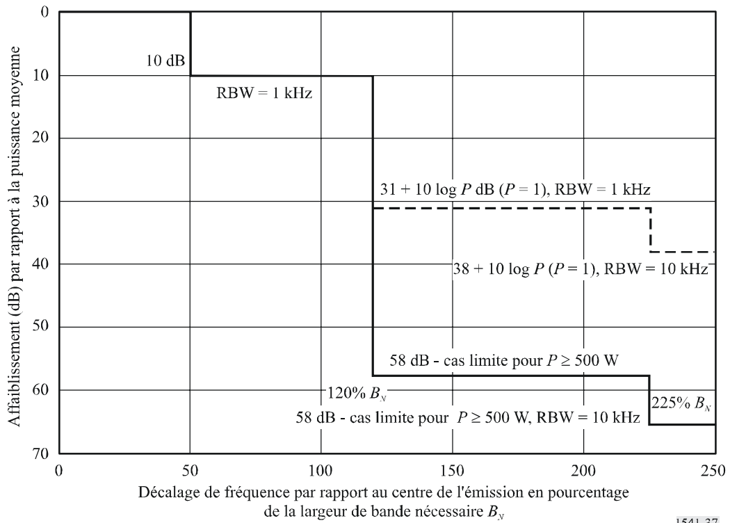
FIGURE 37 Stations fonctionnant au-dessus de 30 MHz dans le cas normal ou dans le cas à bande étroite de la Recommandation UIT-R SM.1539
