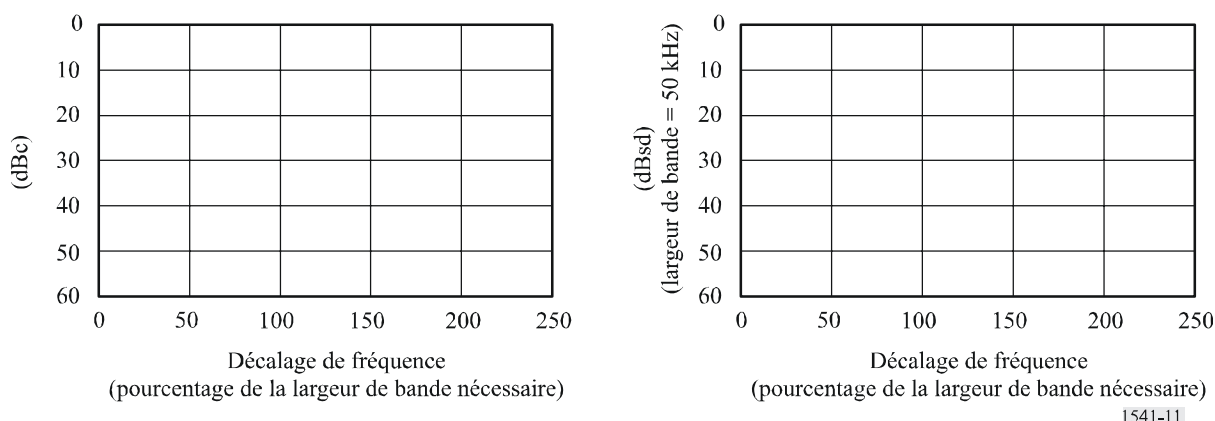
FIGURE 11 Exemples d'un autre étiquetage possible de l'axe des Y pour les gabarits symétriques des émissions hors bande, utilisant les valeurs de l'affaiblissement
