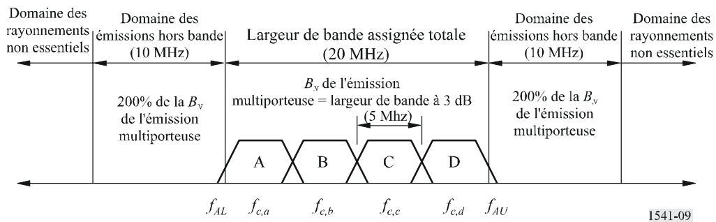
FIGURE 9 Domaine des émissions hors bande et domaine des rayonnements non essentiels dans le cas du système multiporteuse considéré à la Fig. 8
