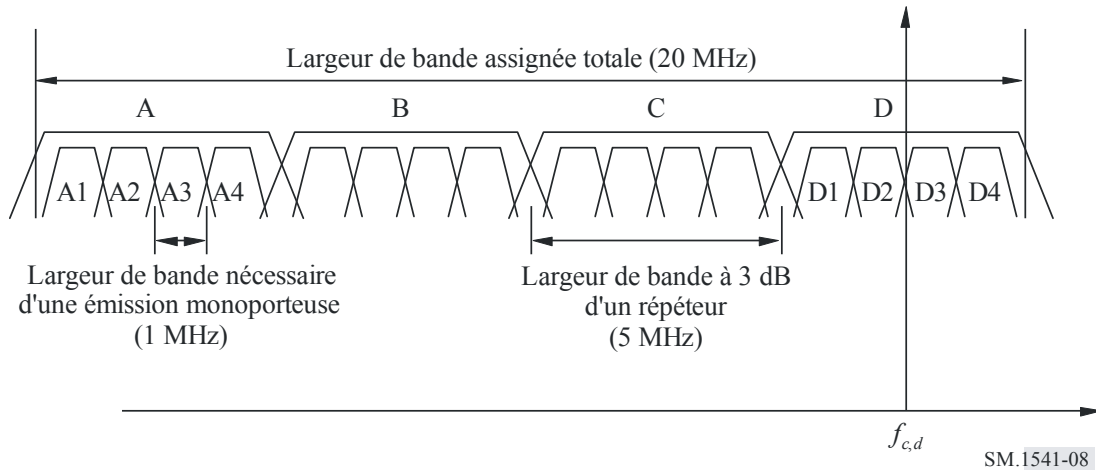
FIGURE 8 Emission multiporteuse avec une largeur de bande à 3 dB de répéteur inférieure à la largeur de bande assignée totale
