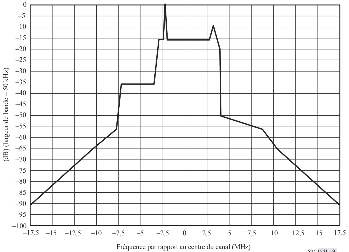
Gabarit de limite spectrale pour la télévision analogique à 7 MHz, modulation négative, BLR de 0,75 MHz (pour P = 39 à 50 dBW)
