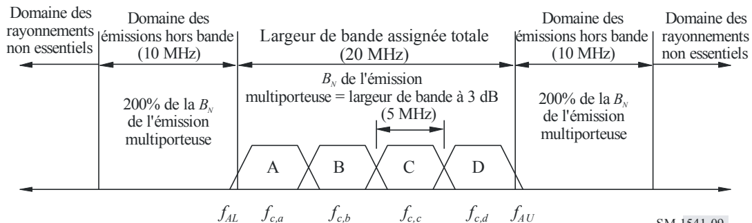
FIGURE 9 Domaine des émissions hors bande et domaine des rayonnements non essentiels dans le cas du système multiporteuse considéré à la Fig. 8
