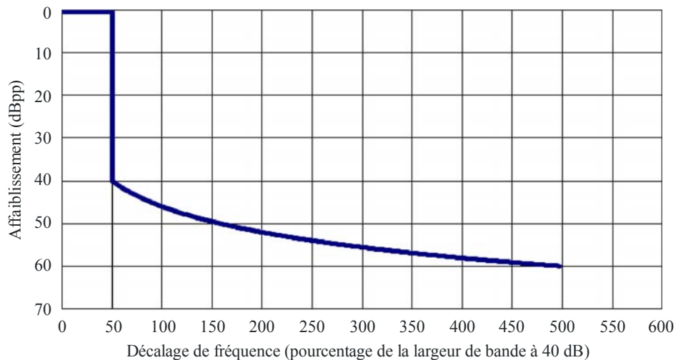
Gabarit des émissions hors bande pour des radars utilisant des formes d'onde entretenues, des formes d'ondes FMCW et des signaux codés en phase
