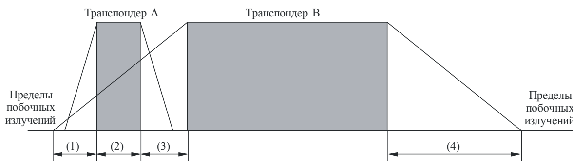
Пример применимости пределов ОоВ для спутникового транспондера (рисунок не в масштабе)
