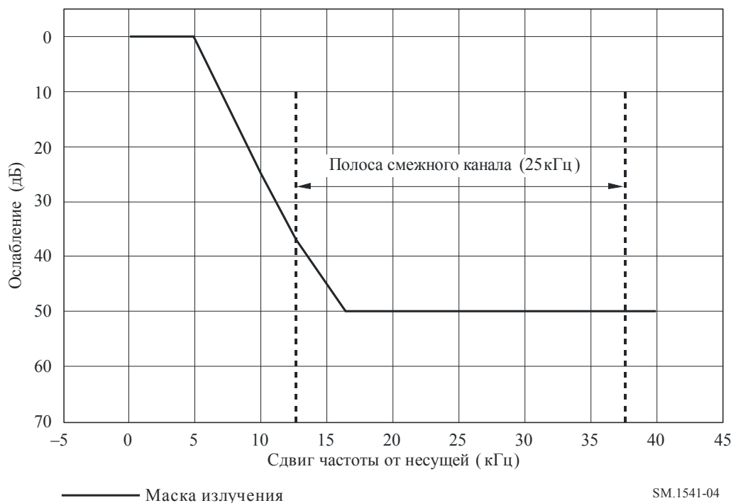
РИСУНОК 4 Маска излучения G (на основе RBW = 300 Гц)
