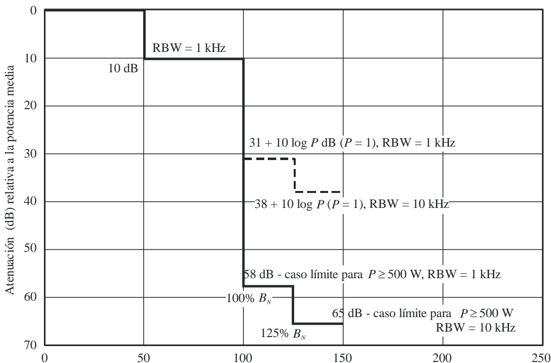
FIGURA 35 Estaciones que funcionan por encima de 30 MHz en el caso de banda ancha de la Recomendación UIT-R SM.1539
