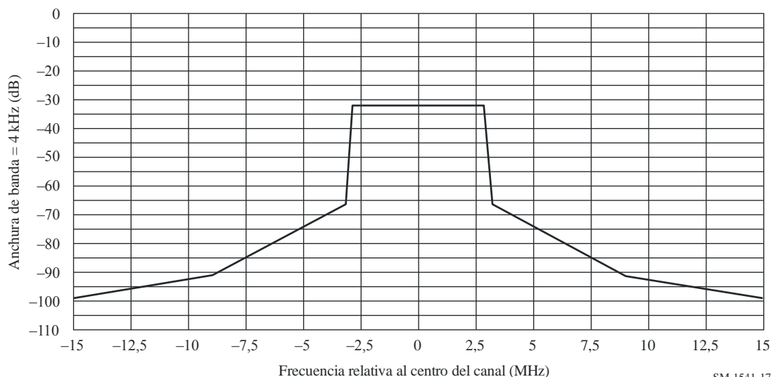
Contorno del límite espectral para la DVB-T de 6 MHz (para P = 39 a 50 dBW)
