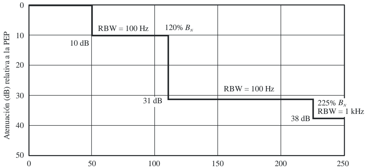
FIGURA 32 Estaciones que funcionan a frecuencias inferiores a 30 MHz en los casos normales o de banda estrecha de la Recomendación UIT-R SM.1539
