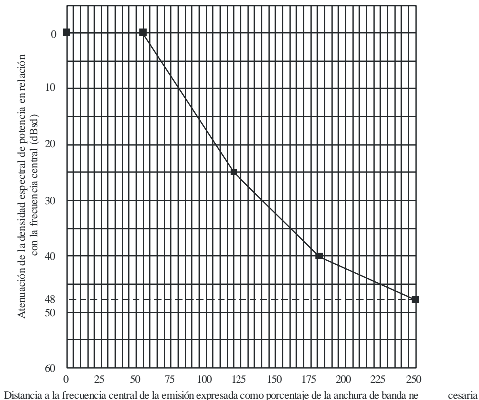
FIGURA 43 Máscaras espectrales genéricas para el servicio fijo digital por debajo de 30 MHz (véase el Cuadro 29)
