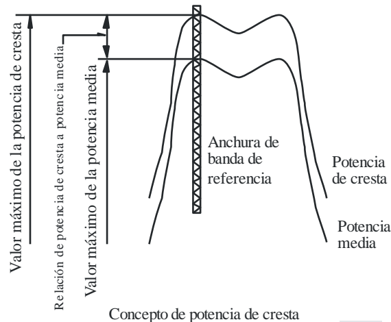
Concepto de potencia de cresta
