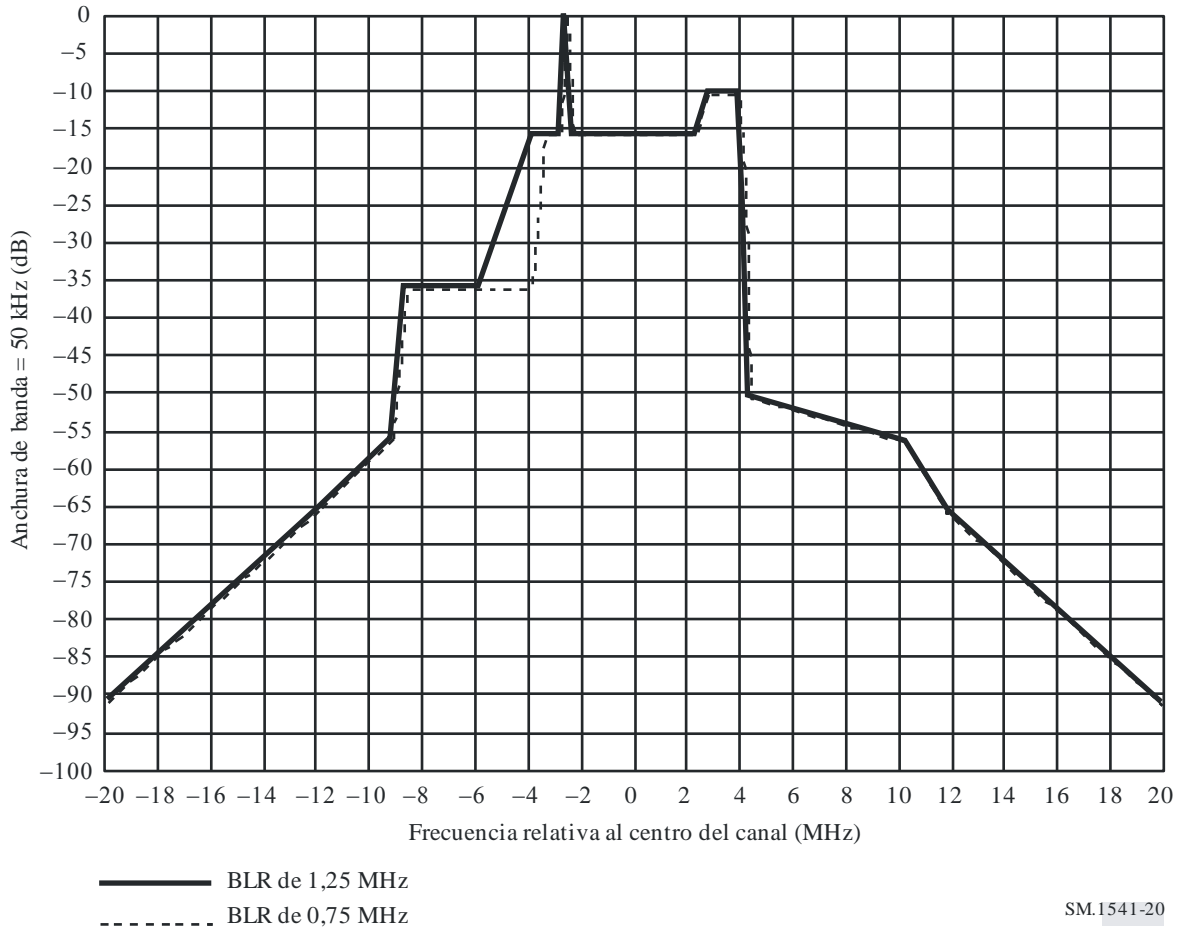
FIGURA 20 Máscara del límite espectral para la televisión analógica de 8 MHz, modulación negativa (para P = 39 a 50 dBW)
