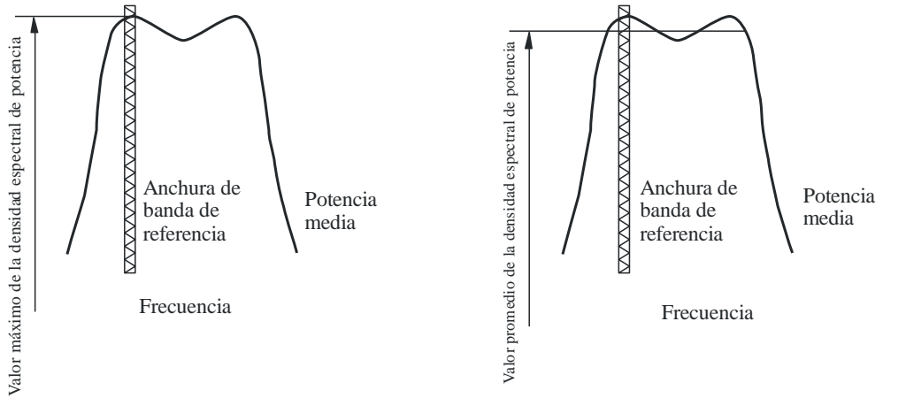
a) Concepto de densidad espectral de potencia máxima
