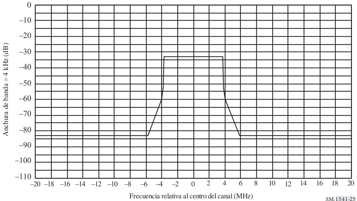
Máscara de límites espectrales para los sistemas ISDB-T de 8 MHz (para P > 39 dBW)
