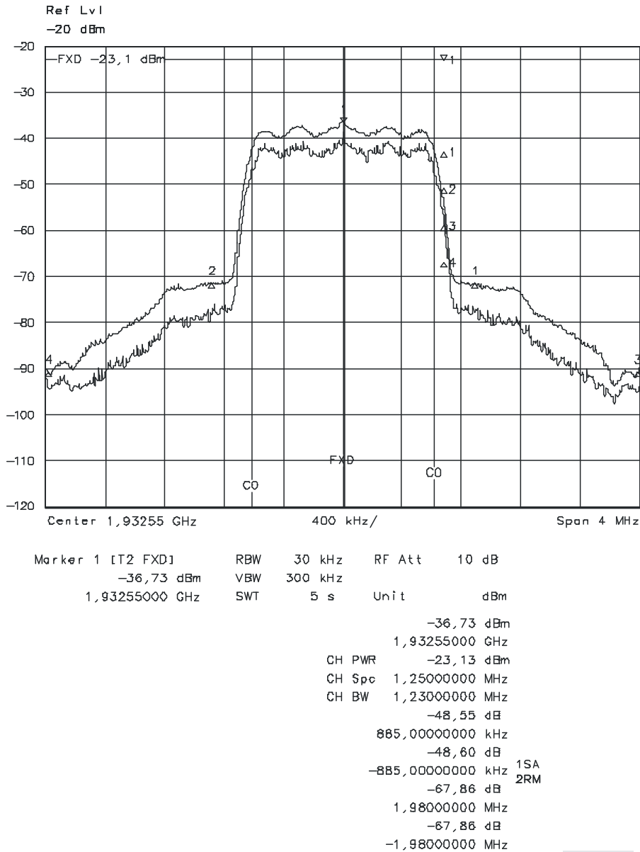
FIGURA 44 Espectro del enlace ascendente de acceso múltiple por división de código (IS95) medido con la función de medición de potencia media verdadera (línea superior) y con promediación de traza (línea inferior)
