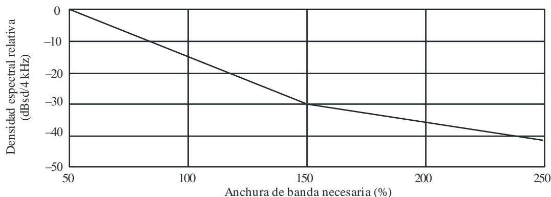
Máscara fuera de banda recomendada para las emisiones de portadora única del servicio de investigación espacial, el servicio de operaciones espaciales y el SETS en los sentidos espacio-Tierra y Tierra-espacio en las bandas entre 1 GHz y 20 GHz
