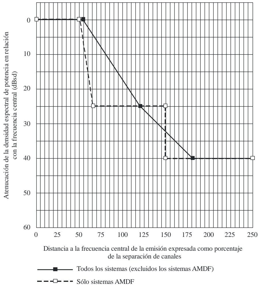
FIGURA 42 Máscaras espectrales genéricas para el servicio fijo digital por encima de 30 MHz (véase el Cuadro 28)
