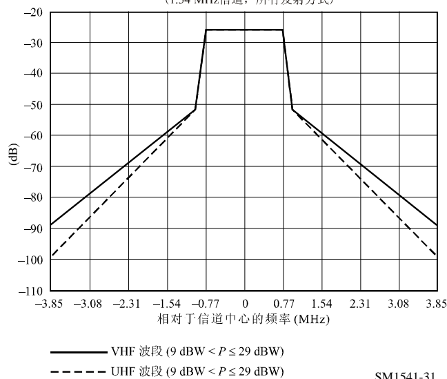
数字系统A的频谱限制掩模 (9 dBW < P ≤ 29 dBW)
