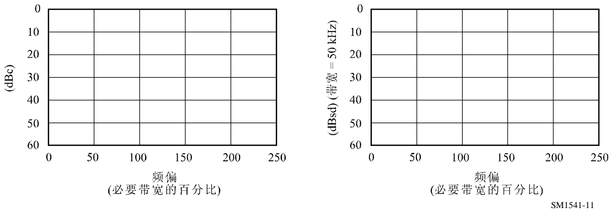
可替代的使用正衰减值的对称OoB掩模Y轴标示的示例
