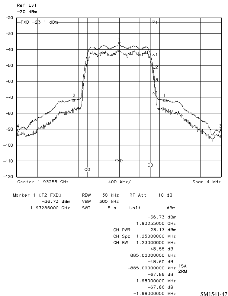
用实际平均功率测量函数（上曲线）和轨迹平均（下曲线）测量的码分多址（IS95）上行频谱
