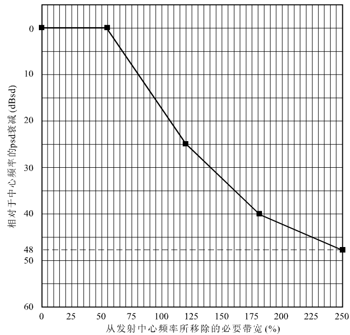
30 MHz以下固定数字业务的常规频谱掩模 (见表32)
