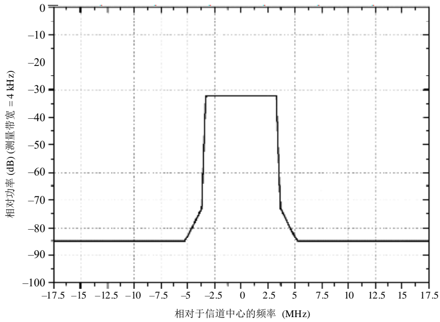
7 MHz DTMB的频谱限值掩膜
