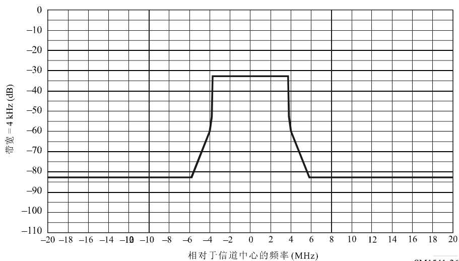
8 MHz ISDB-T的频谱限制掩模 ( P > 39 dBW)
