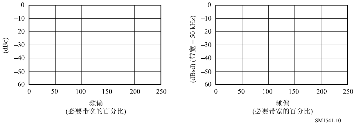
首选的使用相关电平的带外发射的对称Y轴样板标示的示例
