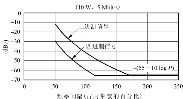
航空遥测带外发射掩模的示例
