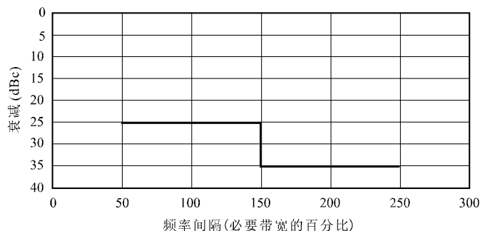
航空和水上移动的OoB掩模
