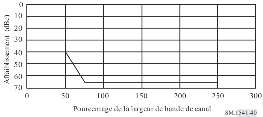
Gabarit des émissions hors bande pour les systèmes à BLU avec compression-extension d'amplitude et à largeur de bande de canal de 5 kHz
