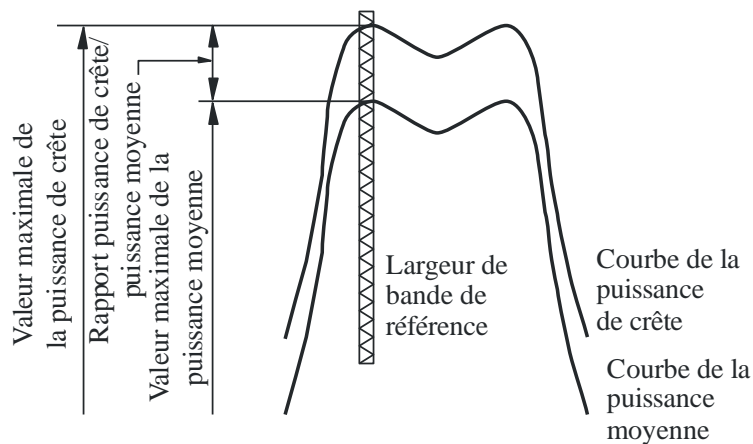
Concept de puissance de crête
