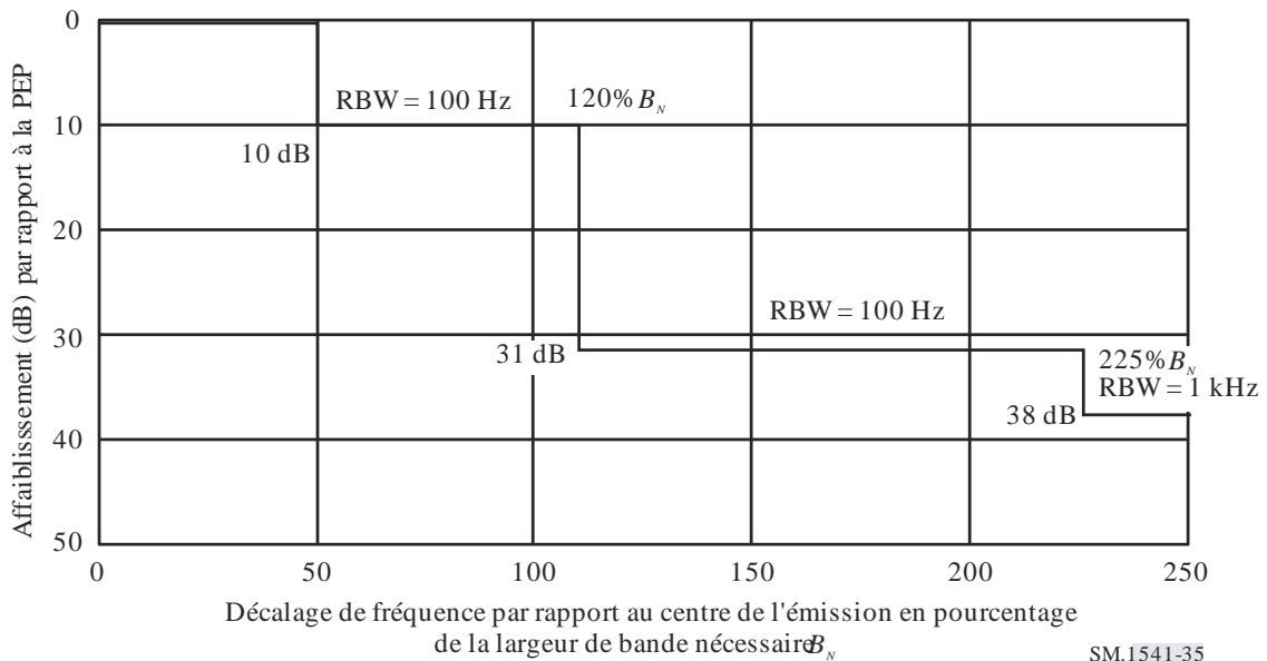
FIGURE 35 Stations fonctionnant au-dessous de 30 MHz dans le cas normal ou dans le cas à bande étroite de la Recommandation UIT-R SM.1539
