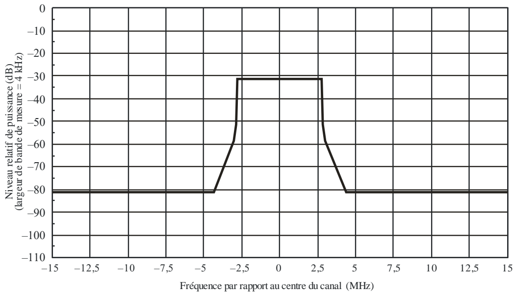
Gabarit de limite spectrale pour les systèmes D (DTMB) à 6 MHz
