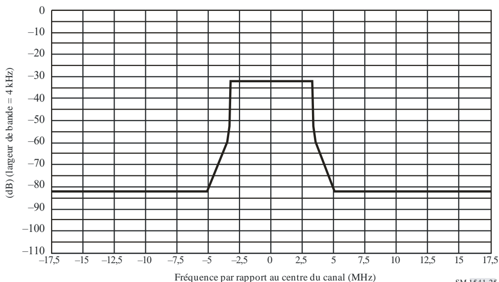
Gabarit de limite spectrale pour les systèmes ISDB-T à 7 MHz (pour P > 39 dBW)
