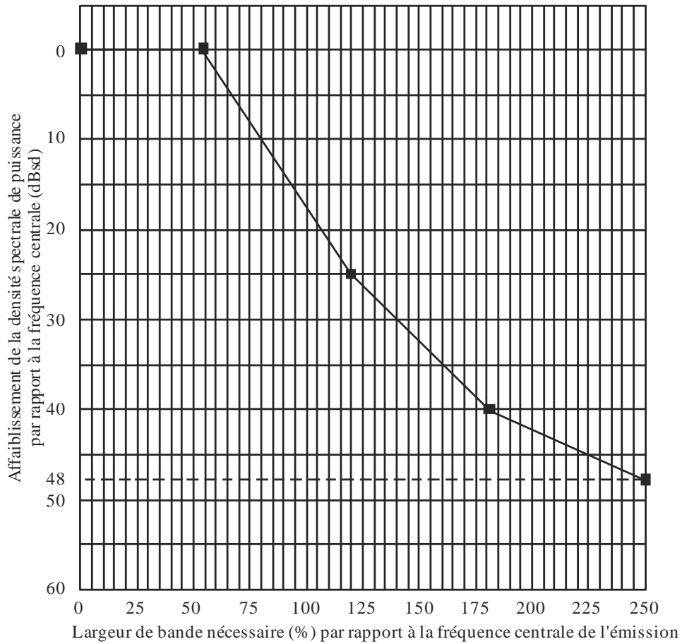
FIGURE 46 Gabarits spectraux génériques pour le service fixe numérique fonctionnant au-dessous de 30 MHz (Voir le Tableau 32)
