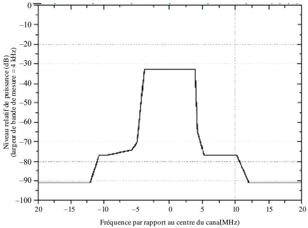
Gabarit de limite spectrale pour les systèmes DTMB à 8 MHz
