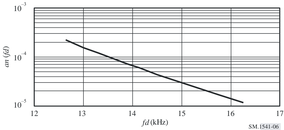
FIGURE 6 Distribution de la puissance de l'émission dans la région du bord proche de la bande adjacente
