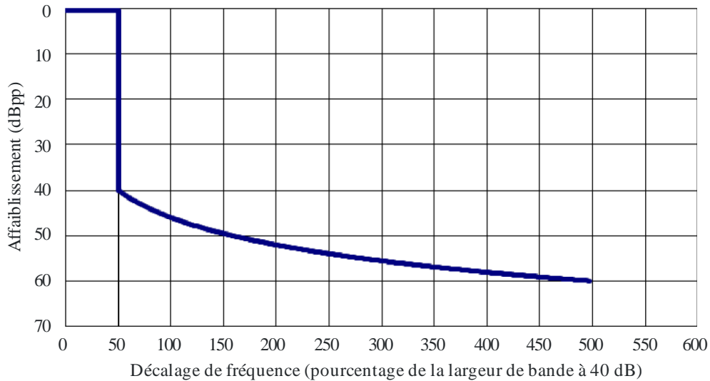
Gabarit des émissions hors bande pour des radars utilisant des formes d'onde entretenues, des formes d'ondes FMCW et des signaux codés en phase
