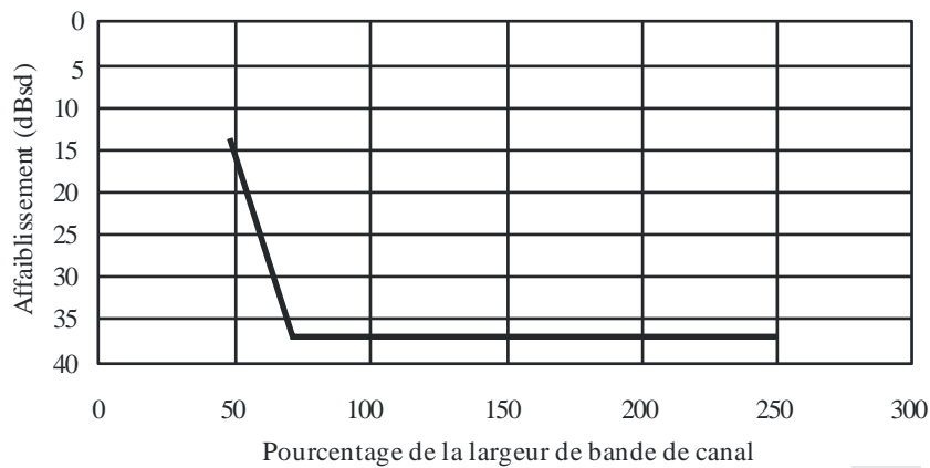
Gabarit des émissions hors bande pour les systèmes mobiles terrestres à largeur de bande de canal de 6,5 kHz
