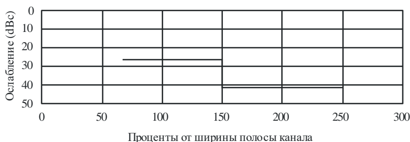
Маска ОоВ для аналоговых сотовых систем с каналами шириной 30 кГц
