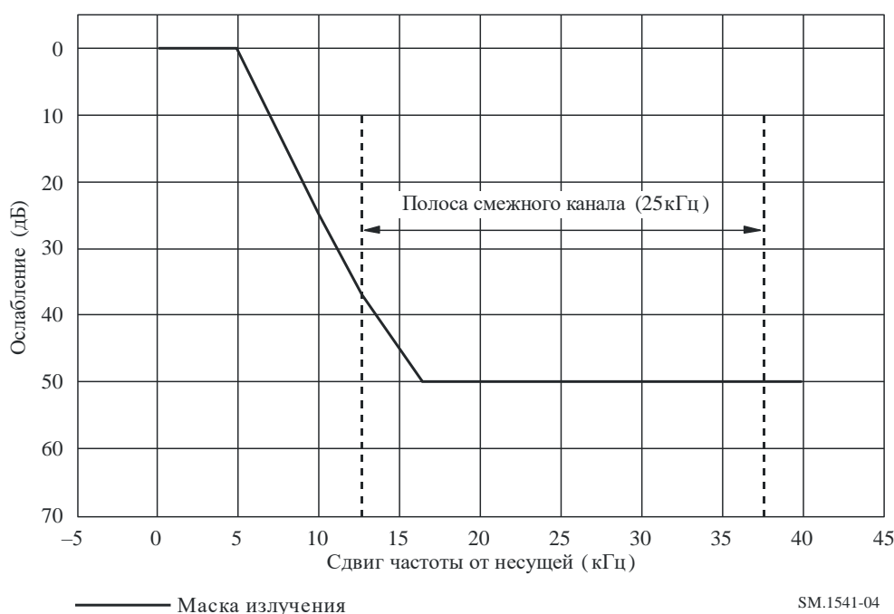
РИСУНОК 4 Маска излучения G (на основе RBW = 300 Гц)
