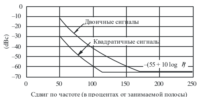
Примеры масок внеполосных излучений для воздушной телеметрии
