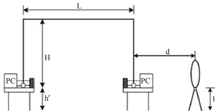
Configuración de la medición desde el lado lateral
