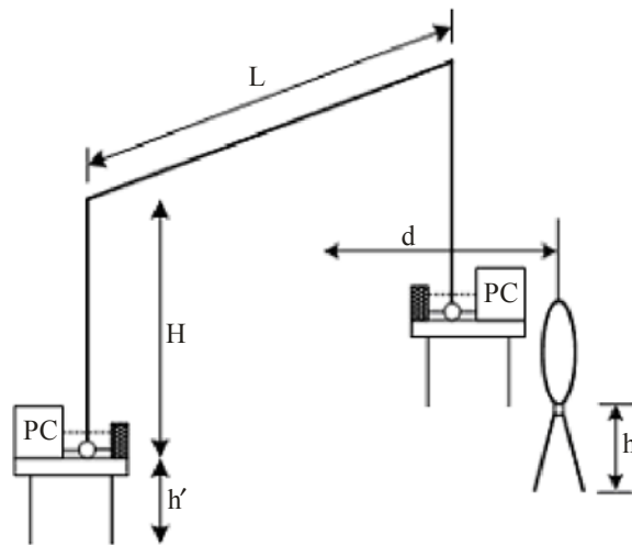
Configuración de la medición desde el lado frontal del PLT
