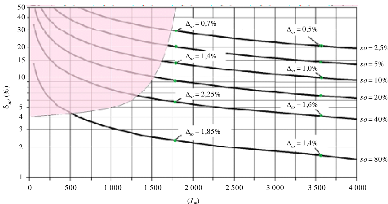
FIGURA 1 Dependencia del error relativo de las estimaciones de ocupación ( \delta_{so} , %) del número de muestras acumuladas ( J_m ) con un nivel de confianza del 95% en canales con señales impulsivas
