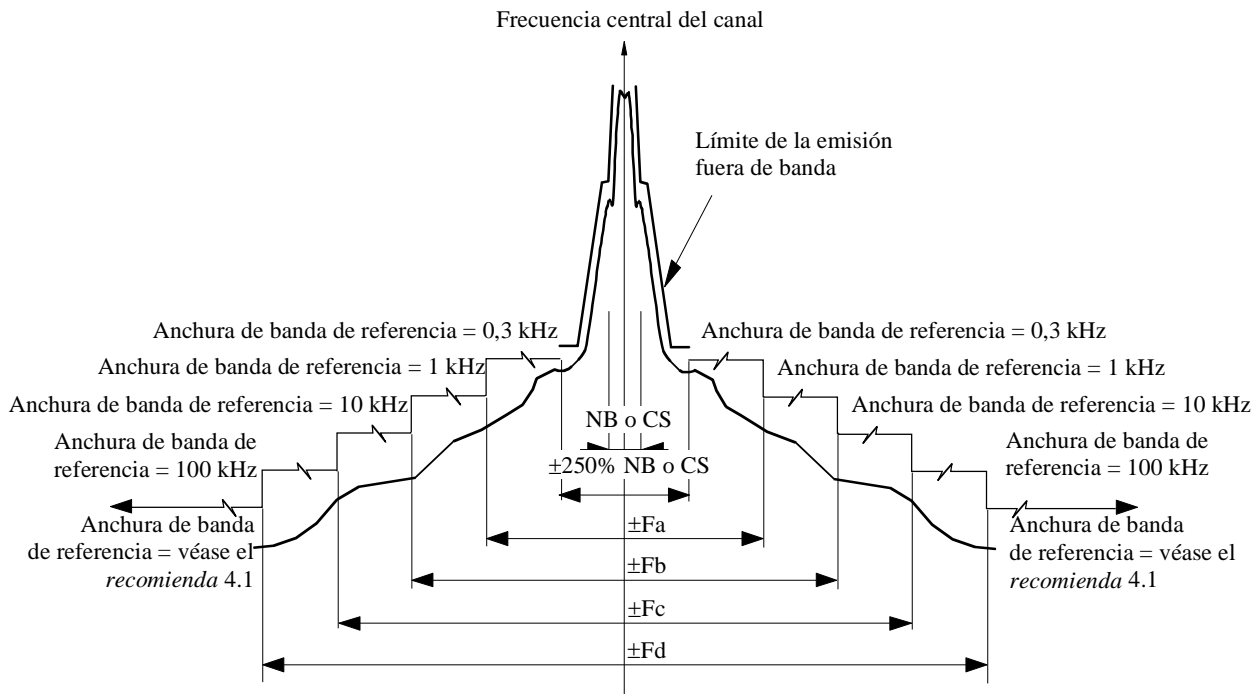
FIGURA 3 Contornos del servicio fijo de Categoría B genéricos para emisiones no deseadas en el dominio no esencial (véase el Cuadro 11)
