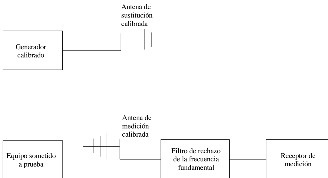
FIGURA 2 Disposición de montaje para la medición de la p.i.r.e. de emisiones no esenciales
