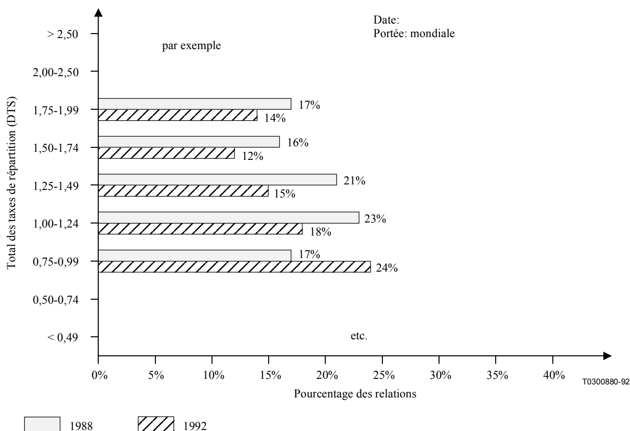
Répartition et variation des taxes de répartition du trafic téléphonique automatique (janvier 1988-janvier 1992)
