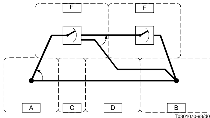
Figure 1/D.170 – Modèle typique d'interconnexion de circuits entre différents pays
