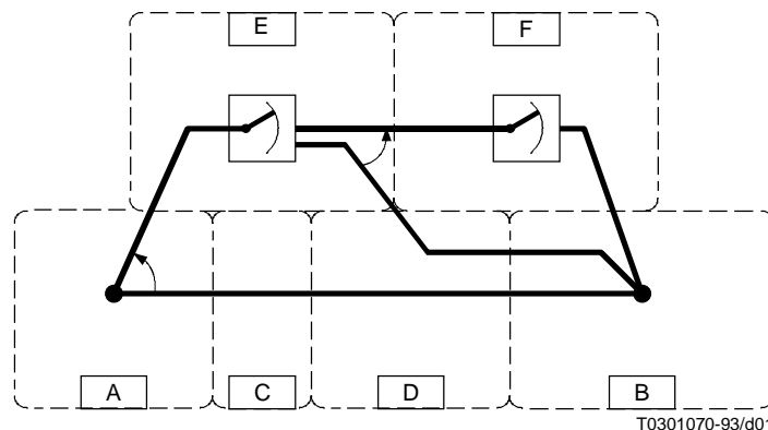
Figura 1/D.170 – Modelo típico de interconexión de circuitos entre diferentes países
