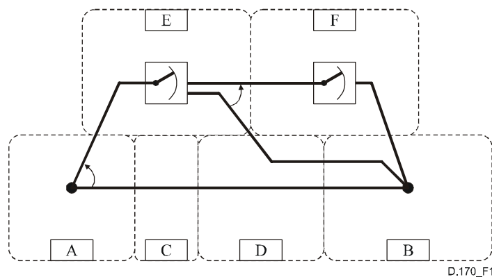
Figure 1/D.170 – Modèle typique d'interconnexion de circuits entre différents pays
