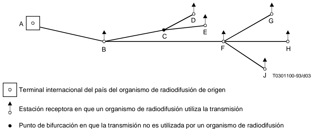
Figura 3/D.180 – Ejemplo de utilización de una red de circuitos internacionales destinados a la realización de una transmisión a destinos múltiples
