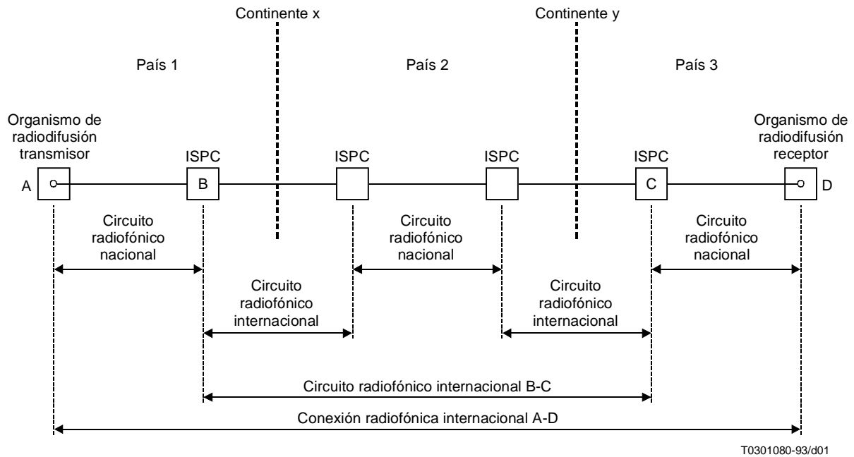
Figura 1/D.180 – Ejemplo de una conexión radiofónica internacional
