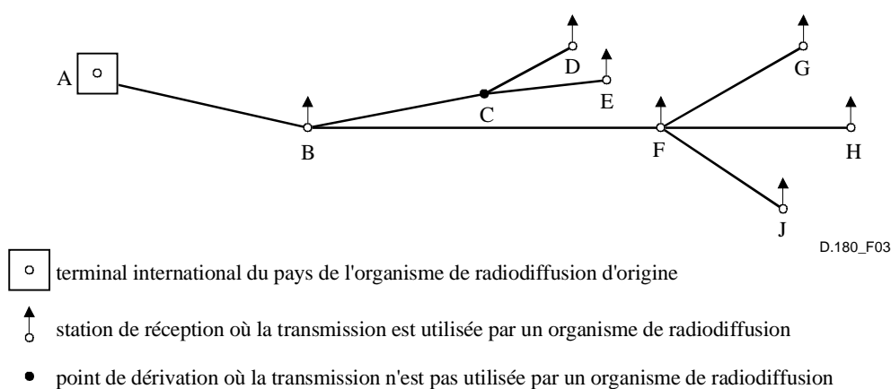
Figure 3/D.180 – Exemple d'utilisation d'un réseau de circuits internationaux destinés à la réalisation d'une transmission à destinations multiples
