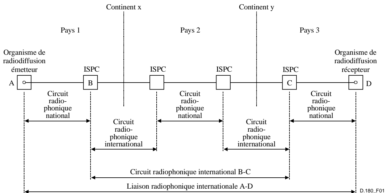
Figure 1/D.180 – Exemple de liaison radiophonique internationale
