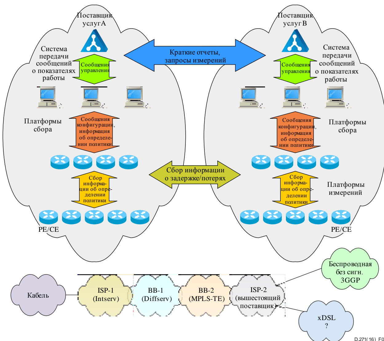
Рисунок 4 – Параметры учета, получаемые на основе данных о взаимодействии QoS
