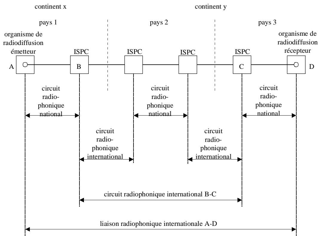
Figure 1/D.4 – Exemple de liaison radiophonique internationale
