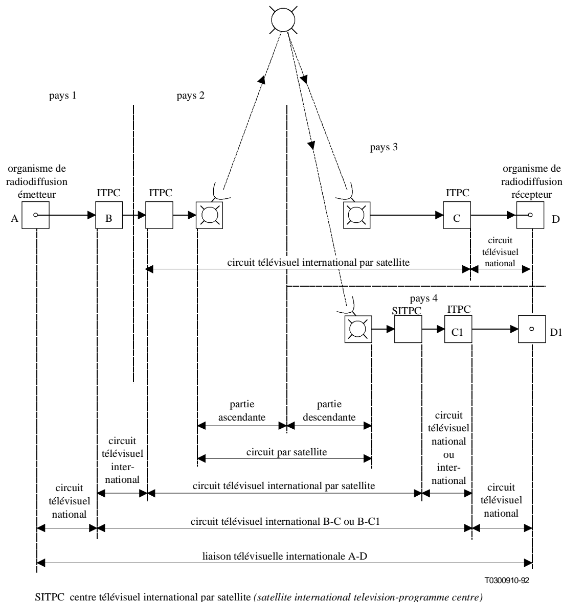
Figure 2/D.4 – Exemple de liaison télévisuelle internationale comprenant un circuit par satellite
