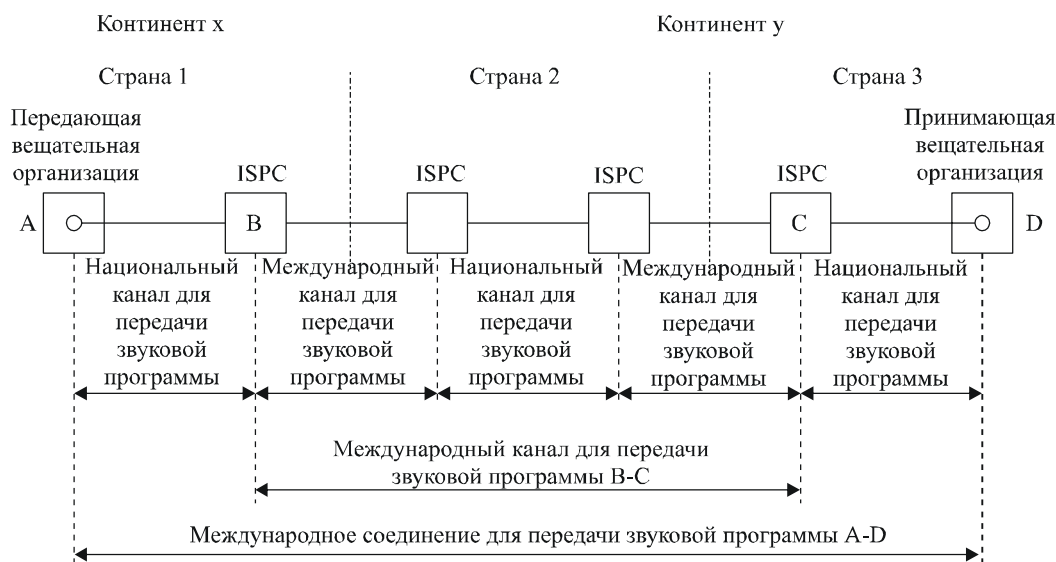
Рисунок 1/D.4 – Пример международного соединения для передачи звуковой программы
