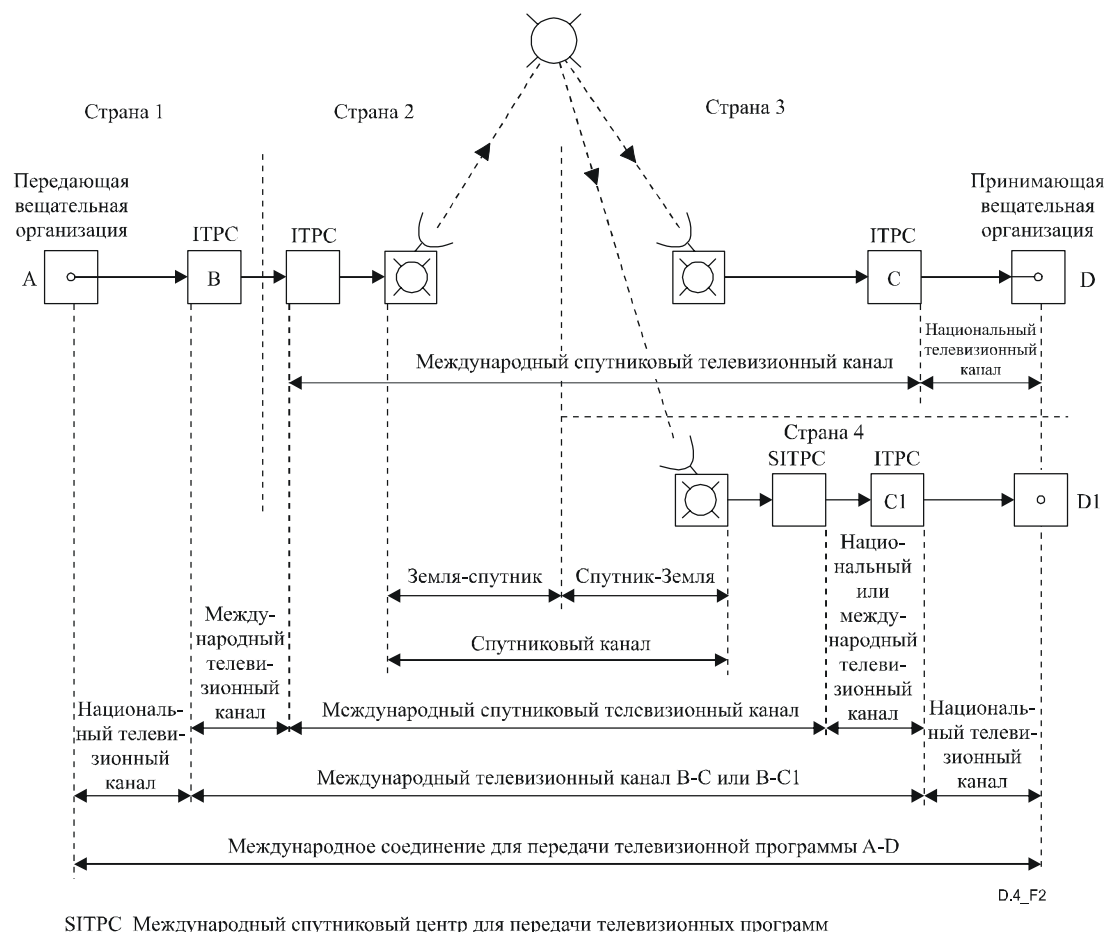
Рисунок 2/D.4 – Пример международного соединения для передачи телевизионной программы с использованием спутникового канала
