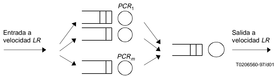
Figura 6-1/E.736 – Espaciador conceptual para m conexiones asignadas a la velocidad de cresta ( \sum PCR_i \leq LR )
