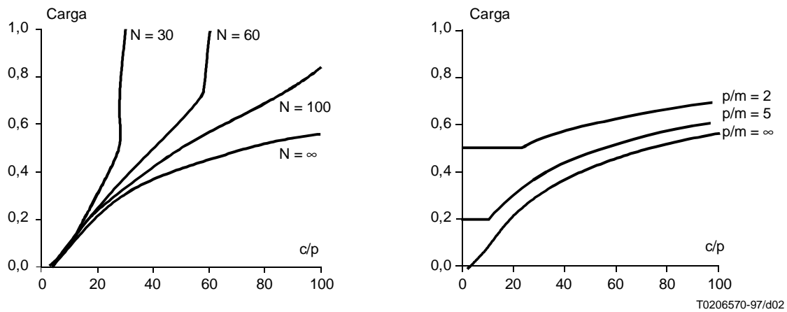
Figura 7-1/E.736 – Carga alcanzable en función de la relación velocidad de enlace/velocidad de cresta (c/p)
