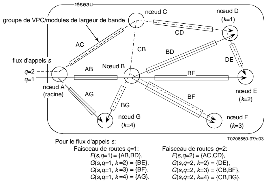
Figure C.1/E.737 – Exemple de faisceaux de routes pour un flux d'appels de type B
