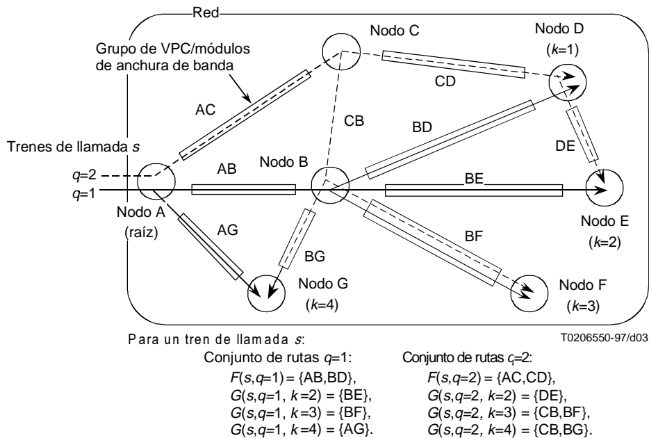
Figura C.1/E.737 – Ejemplo de conjuntos de rutas para un tren de llamadas de tipo B
