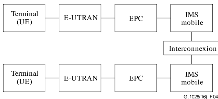
Figure 4 – Modèle de référence hypothétique pour une communication LTE-LTE entre deux réseaux interconnectés
