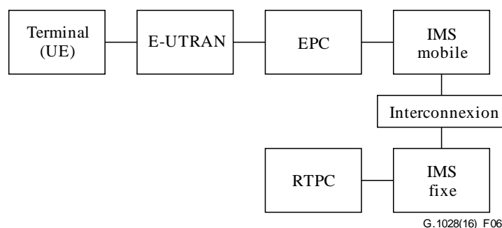
Figure 6 – Modèle de référence hypothétique pour une communication LTE-RTPC
