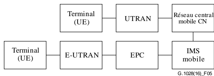
Figure 5 – Modèle de référence hypothétique pour une communication LTE-3G
