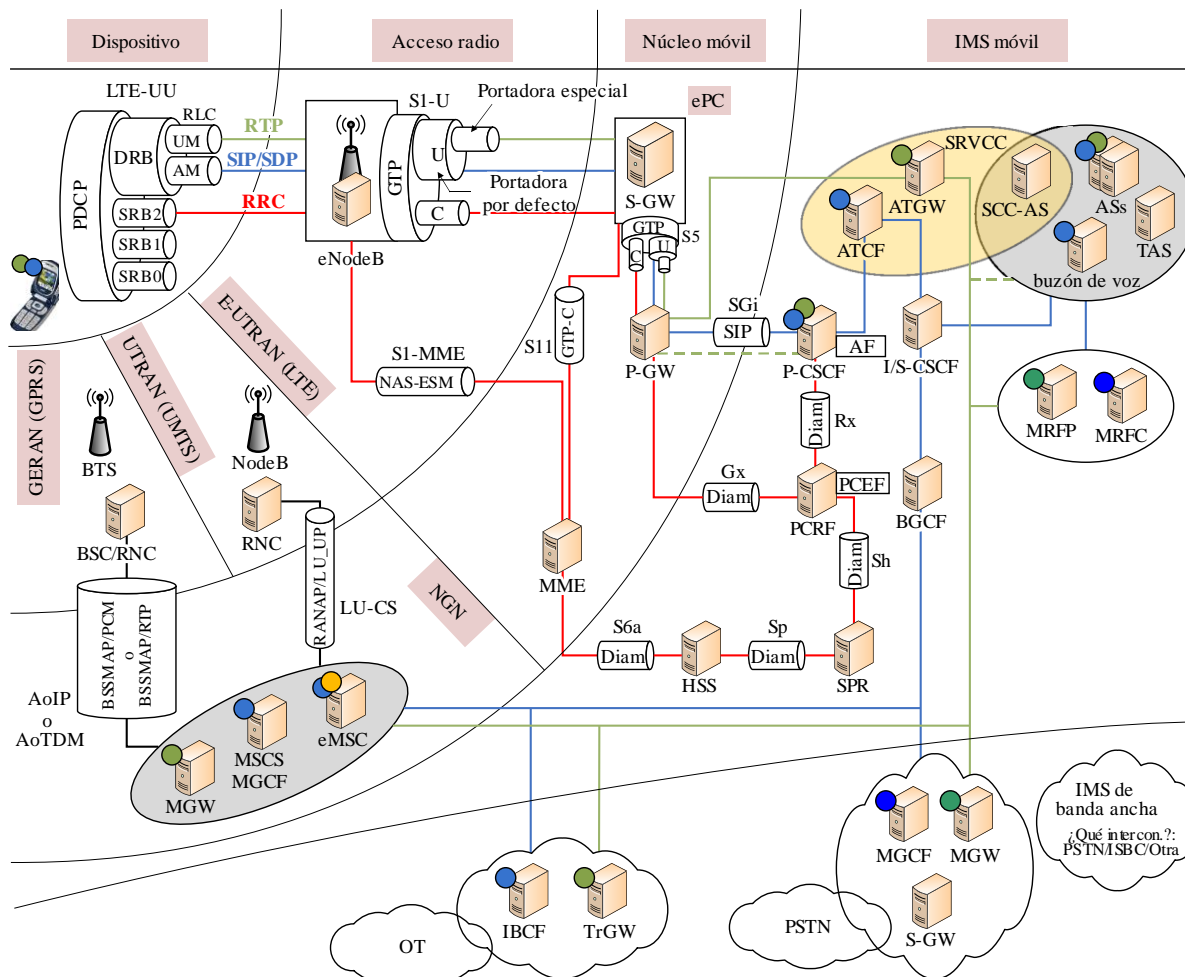
Figura 1 – Arquitectura general de servicios VoLTE
