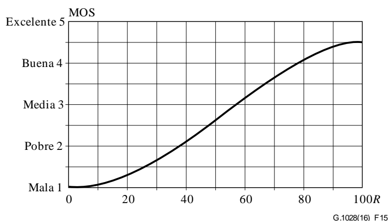
Cuadro 15 – MOS-CQE como función de factor de determinación de índices (fuente: [UIT-T G.107])
