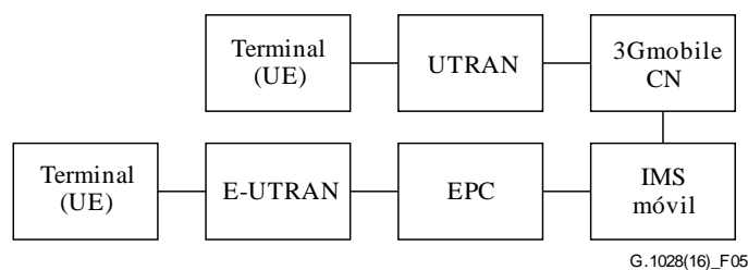
Figura 5 – Modelo de referencia hipotético para una comunicación LTE-3G
