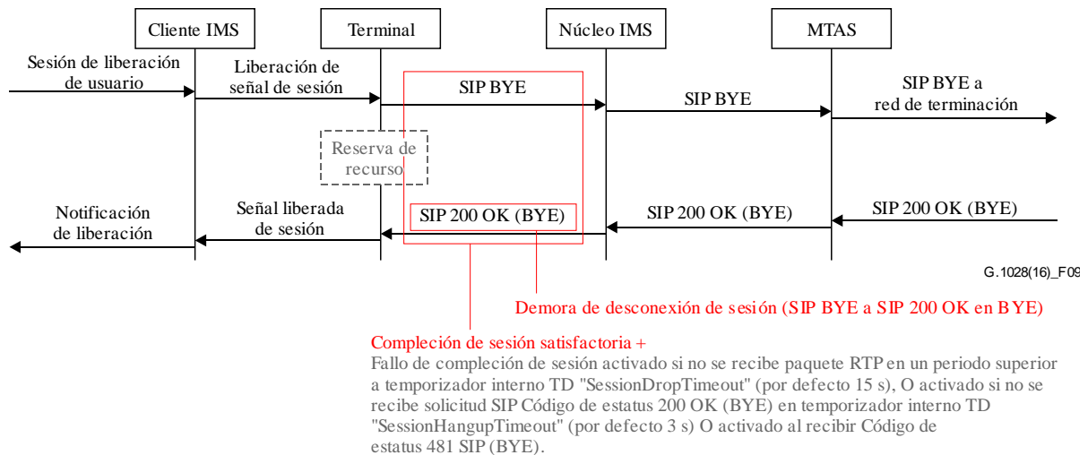
Figura 9 – Flujo de medición de compleción de sesión VoLTE
