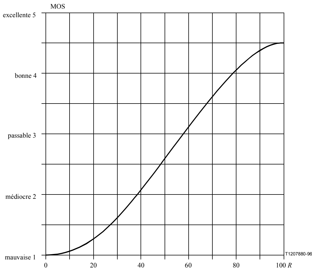
Figure B.2/G.107 – La note moyenne d'opinion MOS en fonction du facteur d'évaluation R
