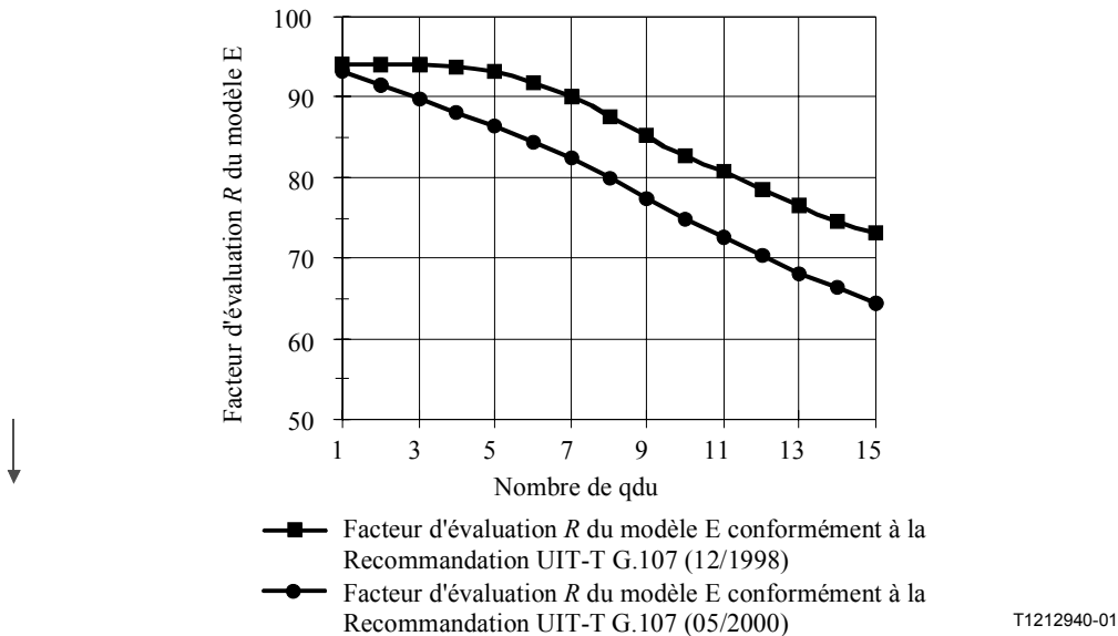
Figure A.1/G.107 – Relation entre le nombre de qdu et le facteur d'évaluation R du modèle E
