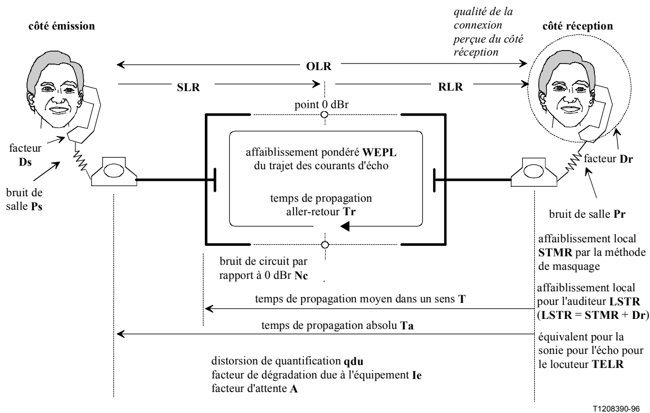
Figure 1/G.107 – Connexion de référence du modèle E
