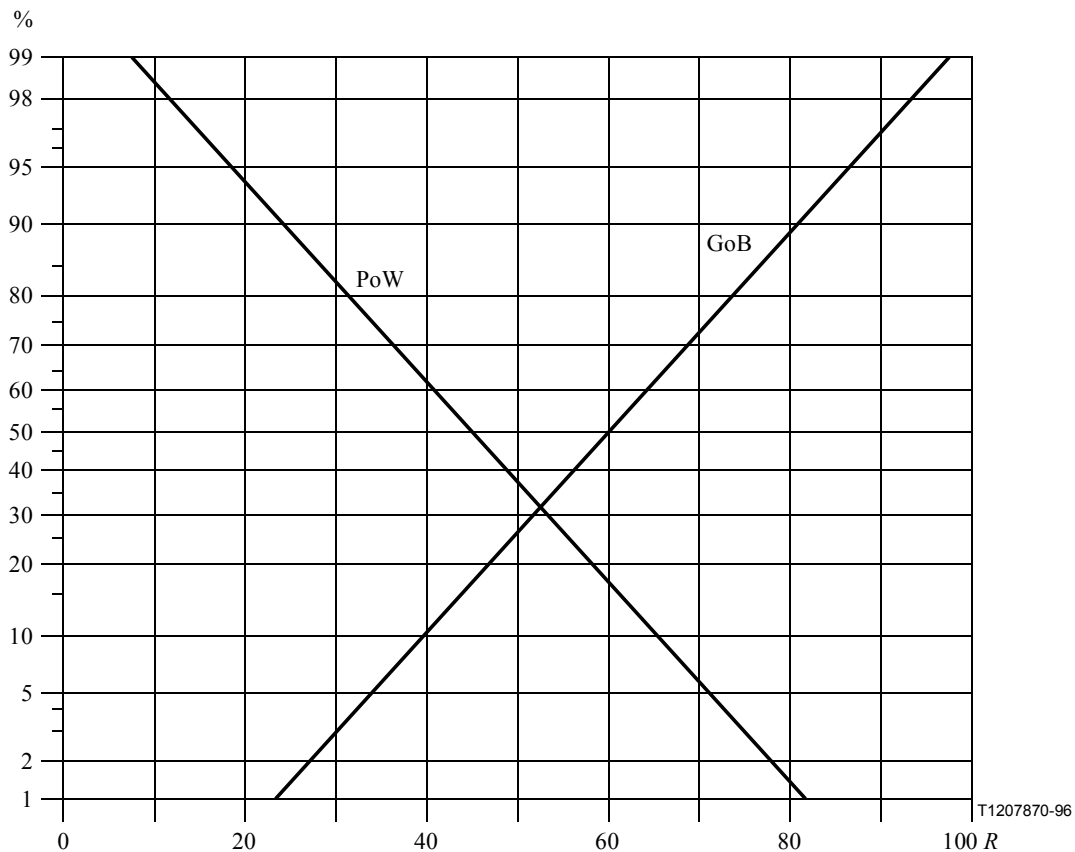
Figure B.1/G.107 – Connexions GoB ("au moins bonnes") et PoW ("au mieux médiocres") en fonction du facteur d'évaluation R
