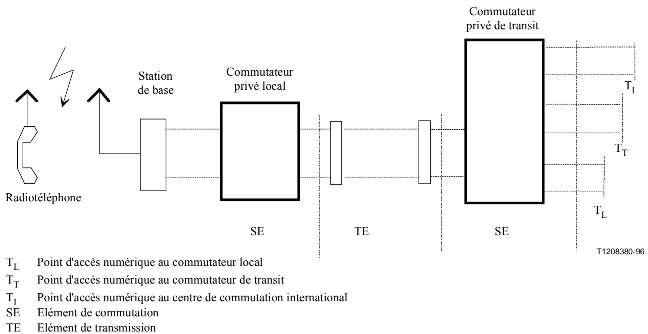
Figure 4/G.175 – Réseau privé associé à un radiotéléphone à connexion numérique
