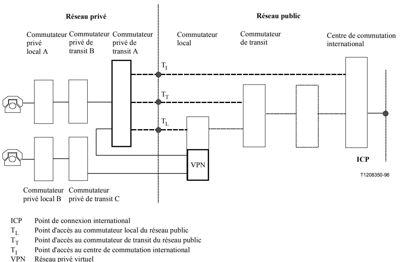
Figure 1/G.175 – Configuration de référence de base pour l'interconnexion de réseaux privés et publics
