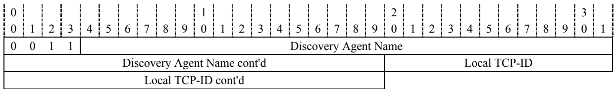
Figure 6/G.7714.1/Y.1705.1 – DA DCN Name Message format
