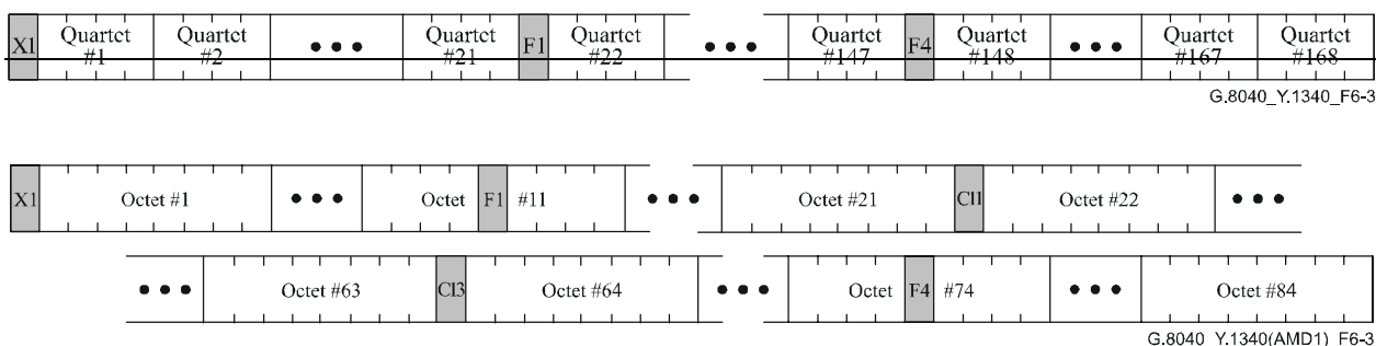
Figure 6-3/G.8040/Y.1340 – Structure des quartets octets pour la sous-trame du signal à 44 736 kbit/s
