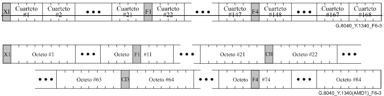
Figura 6-3/G.8040/Y.1340 – Estructura de cuartetos octetos para una subtrama de señal a 44 736 kbit/s
