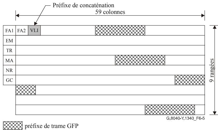
Figure 6-5/G.8040/Y.1340 – Mappage avec alignement des octets des trames GFP dans le signal à 34 368 kbit/s
