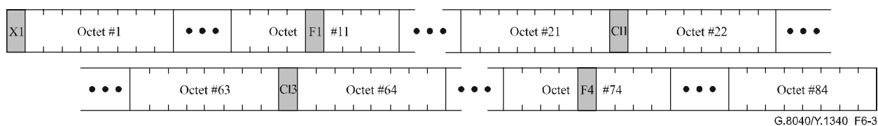
Figure 6-3/G.8040/Y.1340 – Structure des octets pour la sous-trame du signal à 44 736 kbit/s
