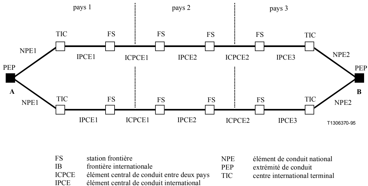
Figure A.2/G.827 – Exemple de conduit avec topologie redondante
