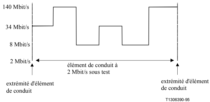
Figure B.1/G.827 – Exemple d'élément de conduit ayant comme support des sections numériques d'ordre supérieur
