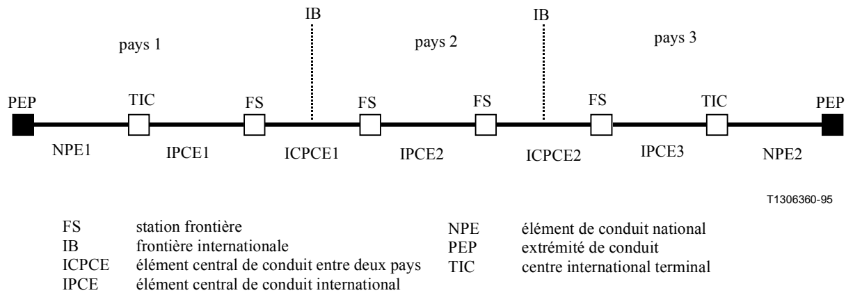
Figure A.1/G.827 – Exemple de conduit avec topologie linéaire
