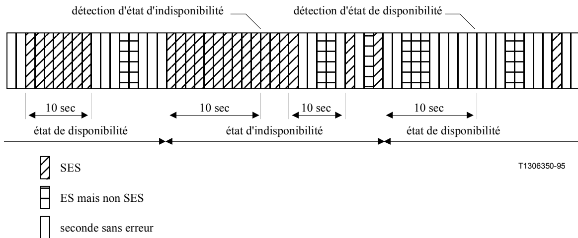
Figure 4/G.827 – Transition entre les états de disponibilité et d'indisponibilité
