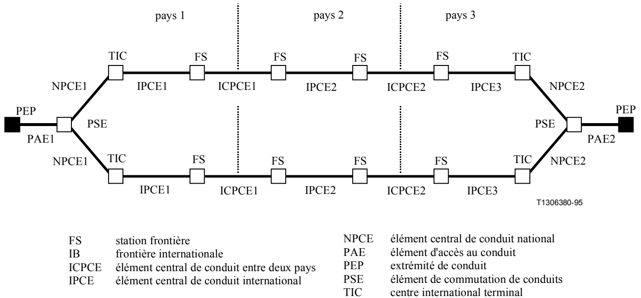
Figure A.3/G.827 – Exemple de conduit comportant à la fois une topologie linéaire et une topologie redondante
