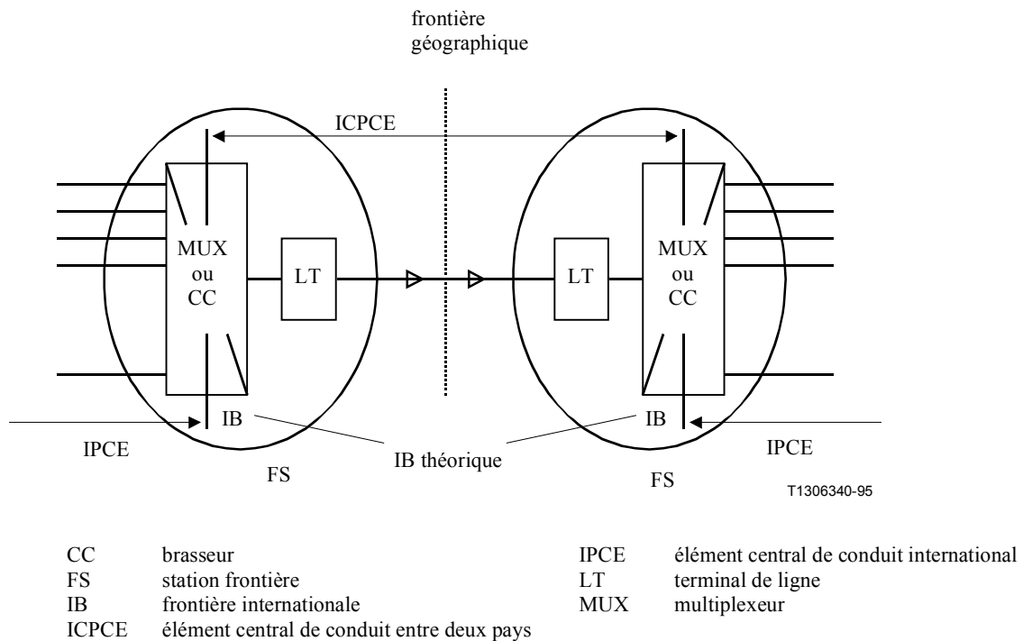
Figure 3/G.827 – Exemple d'élément central de conduit entre deux pays (ICPCE)
