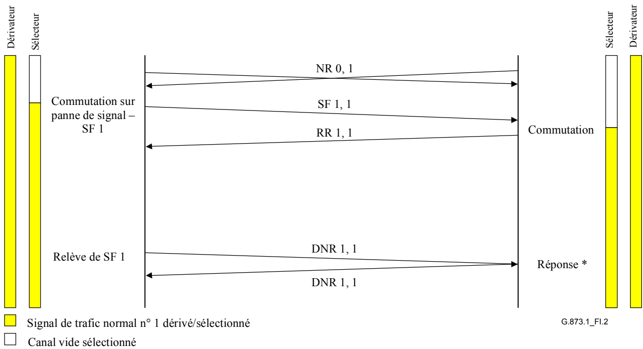
Figure I.2/G.873.1 – Exemple de flux de messages APS pour commutation doublée dans les deux sens
