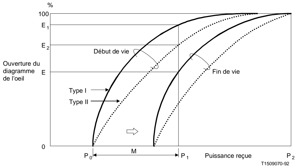
FIGURE III-1/G.957 Caractéristiques du diagramme de l'oeil
