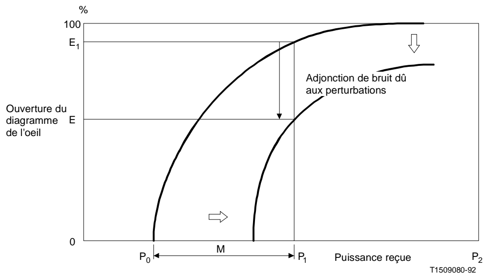
FIGURE III-2/G.957 Ouverture du diagramme de l'oeil due aux perturbations entre les symboles
